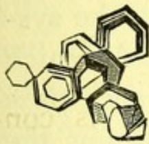
Fig. 2. Cystin.
