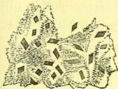
Fig. 8. Hæmin Crystals.
