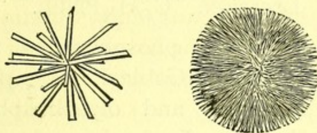
Fig. 3. Tyrosin.
