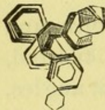
Fig. 14. Cystin.
