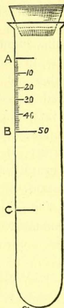
Fig. 9.
