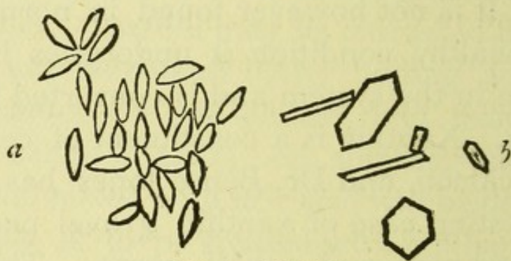
Fig. 5. Xanthin.
