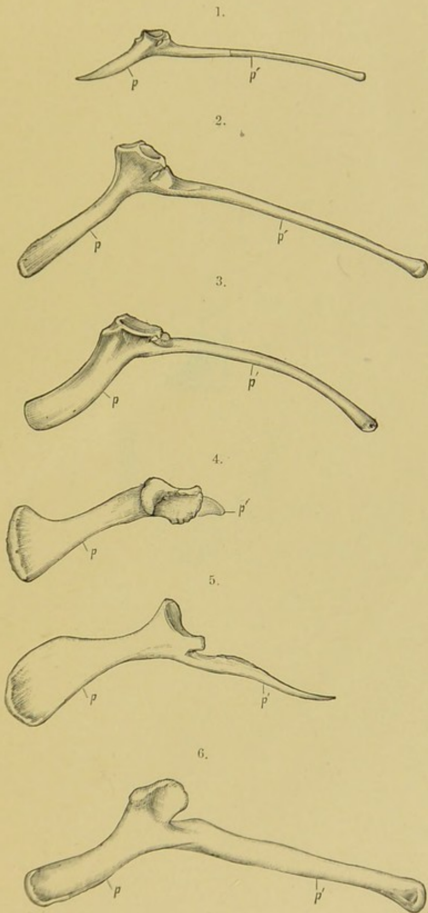
PUBES OF PREDENTATE DINOSAURIA.
