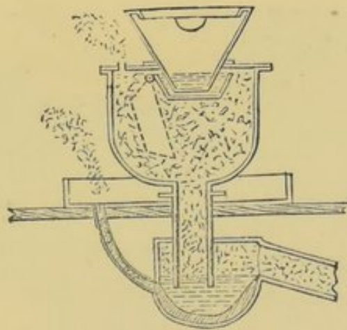
Pan Water-closet.
