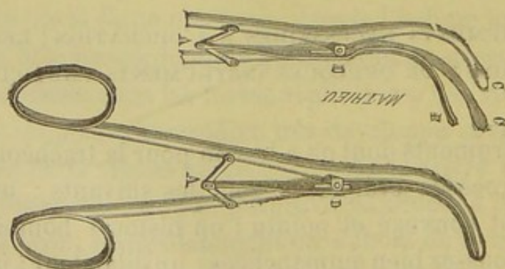
Fig. 1. — Dilatateur de Laborde.
