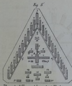
Plan de l'Hôpital Lincoln à Washington
