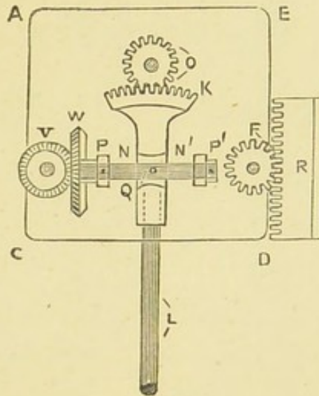
FIG. 15.—Sectional plan.
