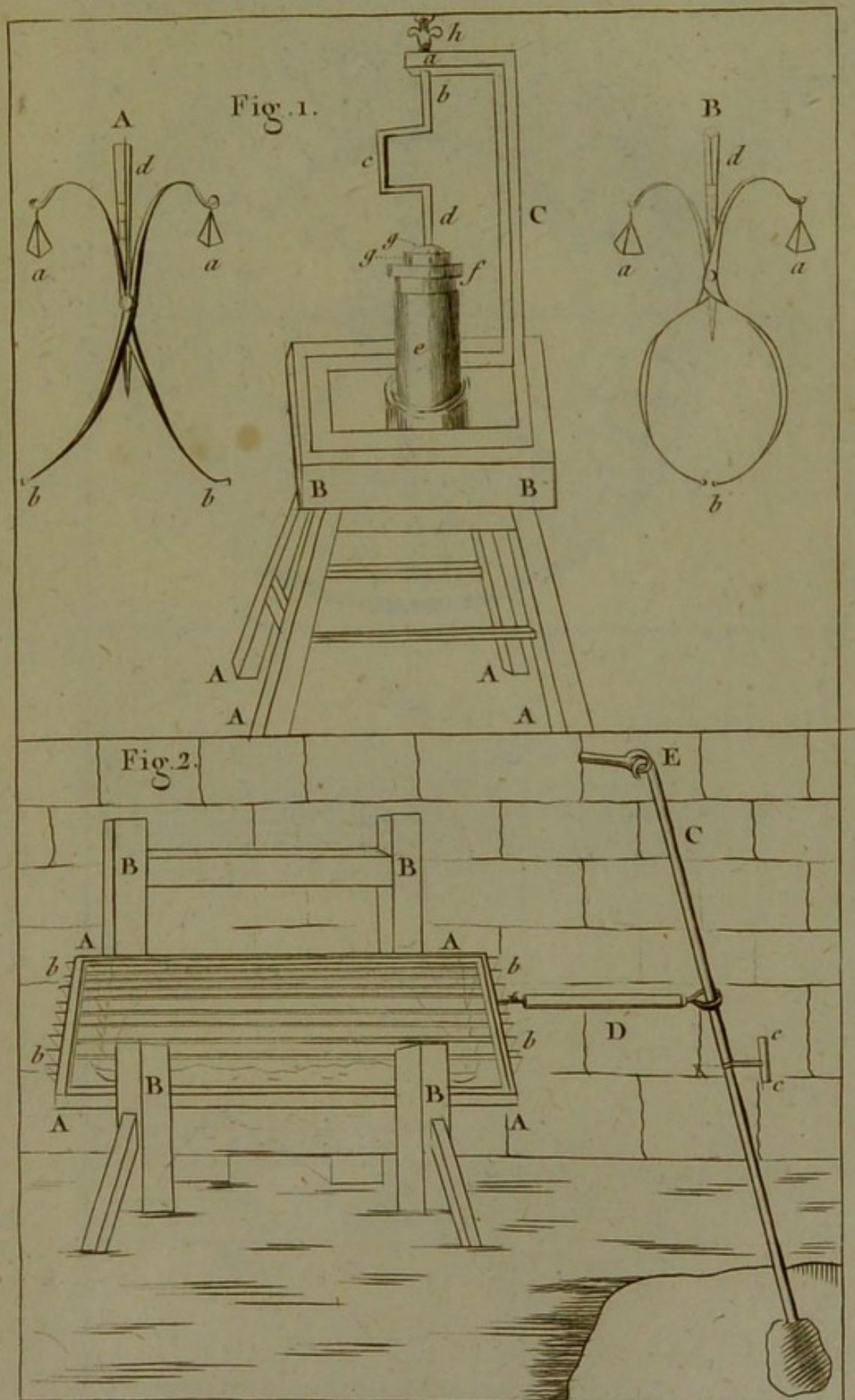
Fig. 1. Moulin à creuser les Vases de Marbre. &c.
