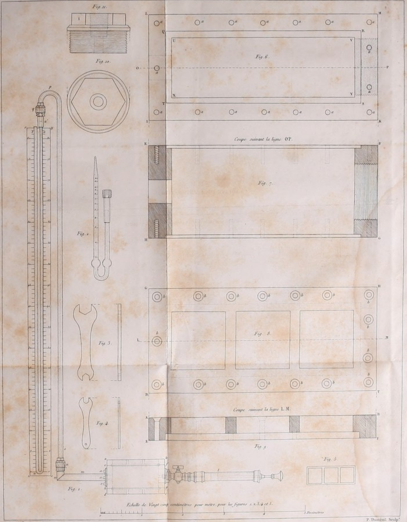
PORTE-OBJET PNEUMATIQUE.
