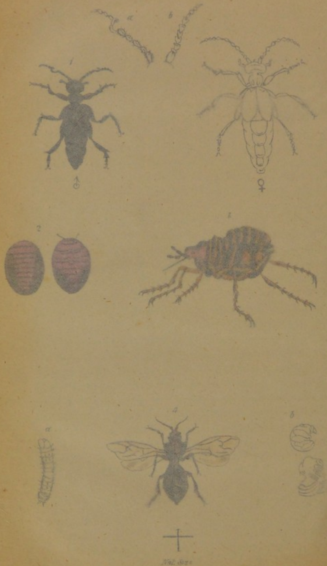
2. Coccus cacti .
