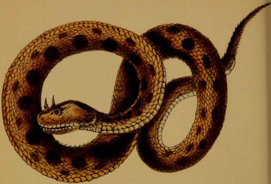
Cerastes vulgaris.
