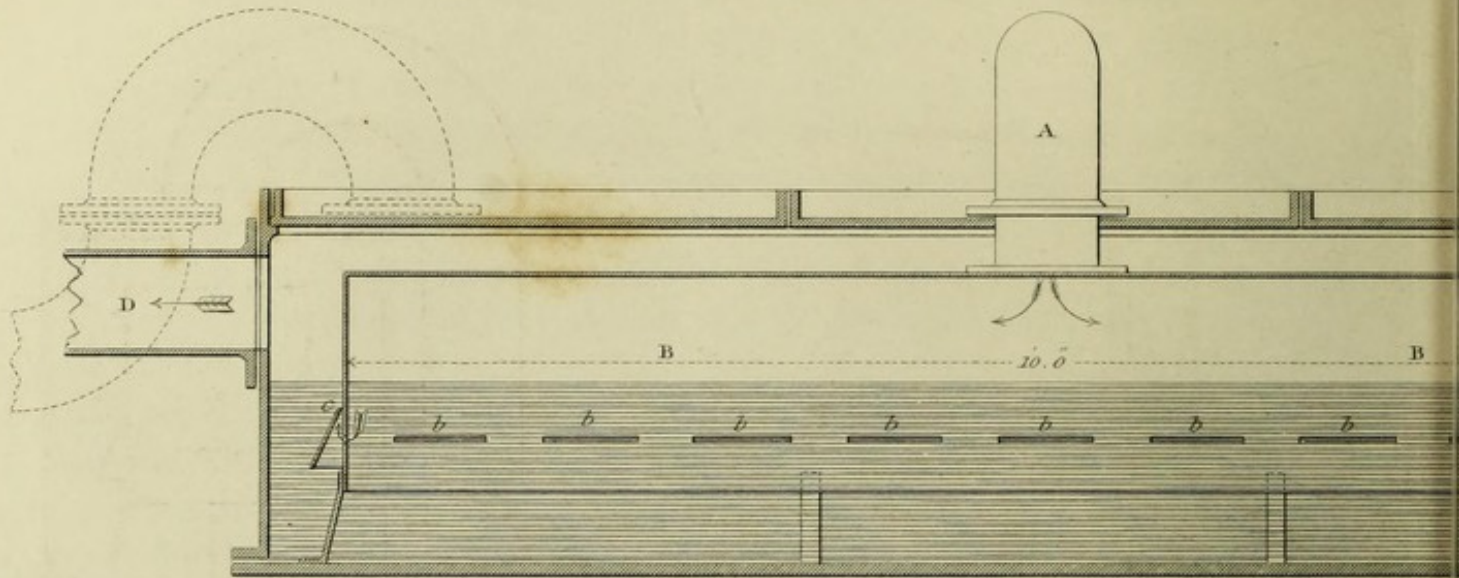
Longitudinal Section.
