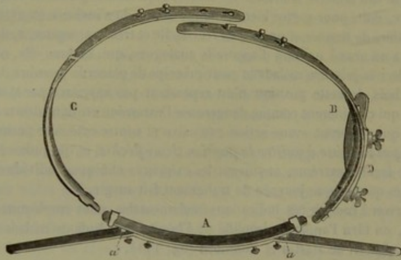
FIG. 172. — Appareil de Ferd. Martin. — Partie de la contre-extension. Ceinture désarticulée.
