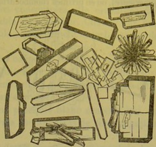
Fig. 77. — Créatine.
