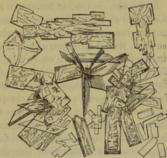
Fig. 51. — Acide benzoïque.
