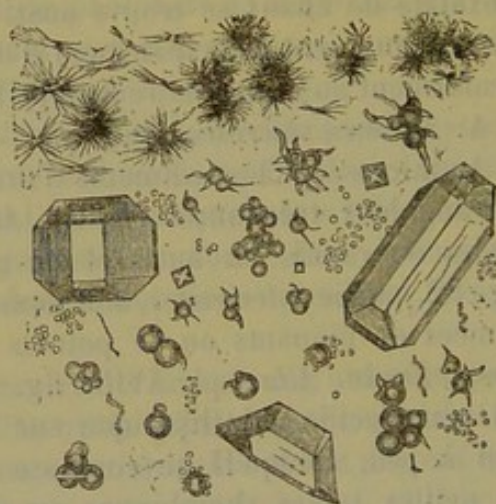
Fig. 93. — Urate d'ammoniaque avec phosphate ammoniaco-magnésien en gros cristaux et octaédres d'oxalate de chaux (sédiment d'une urine alcaline, dans lequel on voit aussi des globules hyalins de ferment urinaire et quelques vibrions).
