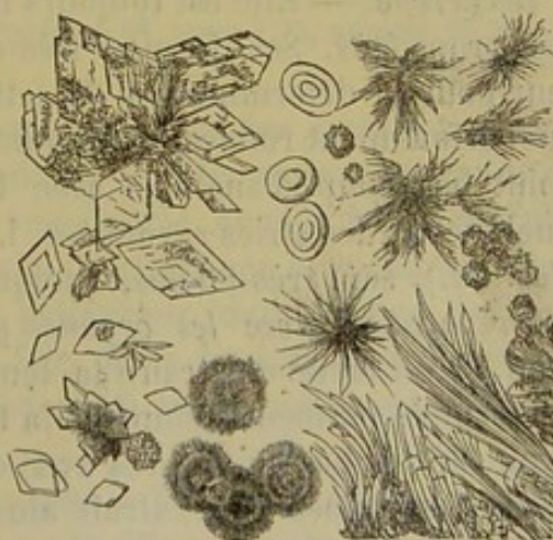
Fig. 81. — Leucine (différentes formes cristallines).
