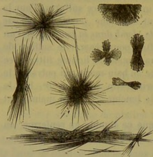
Fig. 82. — Tyrosine.
