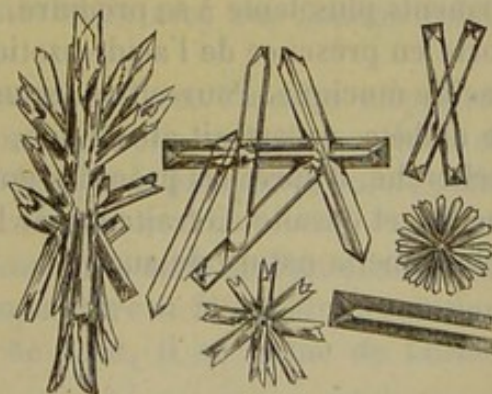
Fig. 48. — Galactose.
