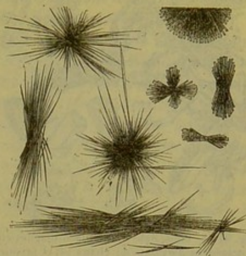
Fig. 90. — Tyrosine.
