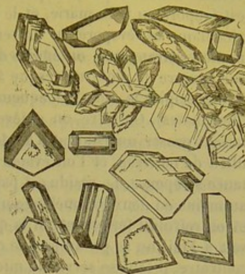
Fig. 67. — Oxalate d'urée.
