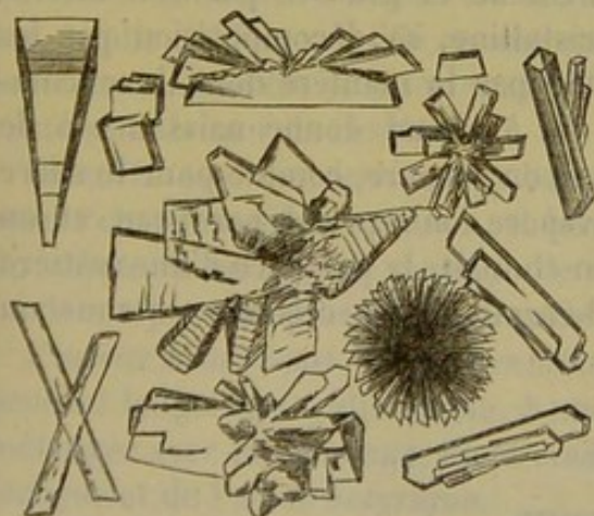
Fig. 47. — Sucre de lait ou lactose.
