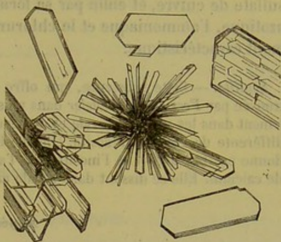
Fig. 49. -- Inosite.
