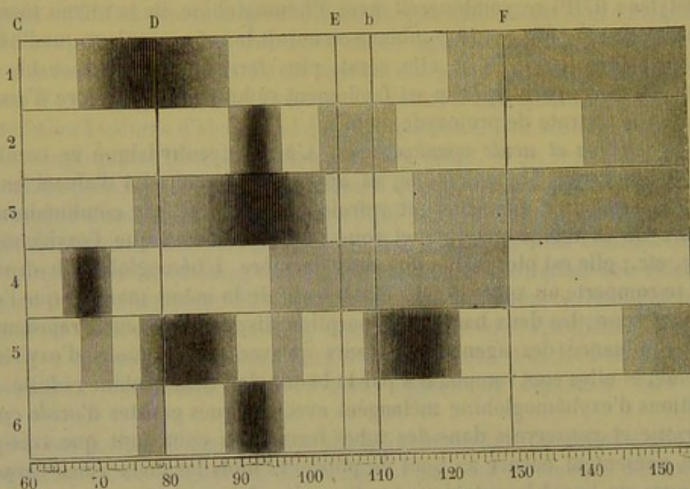
Fig. 44. — Spectres de l'hématine.
