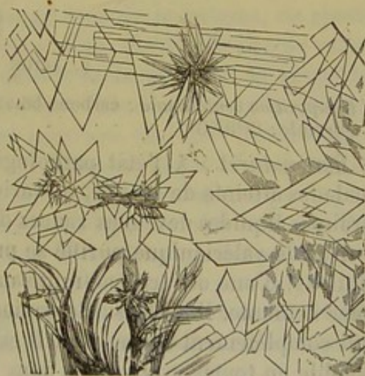
Fig. 50. — Butyrate de baryte.
