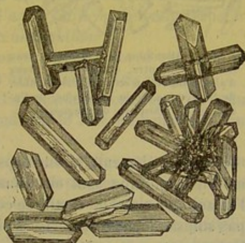
Fig. 75. — Allantoïne pure préparée avec l'acide urique.
