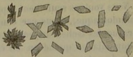
Fig. 125. — Cristaux d'hémine.
