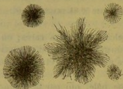
Fig. 70. — Azotate d'argent et de xanthine.
