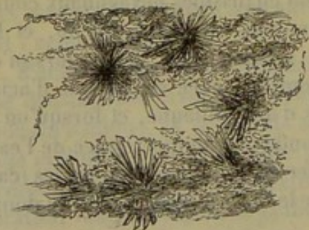
Fig. 58. — Urate de soude d'un tophus arthritique.
