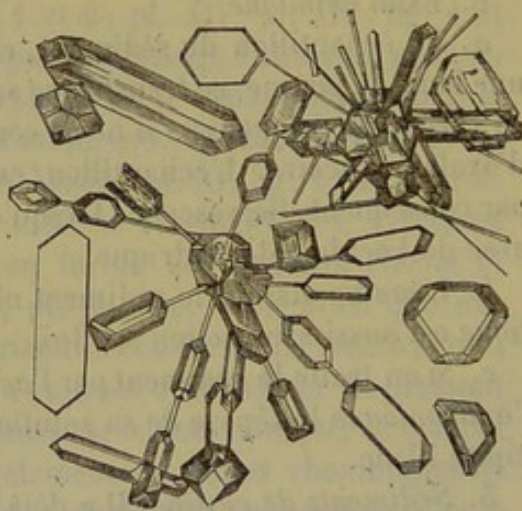
Fig. 89. — Acide hippurique.
