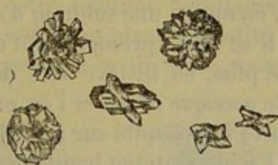
Fig. 69. — Azotate de xanthine.
