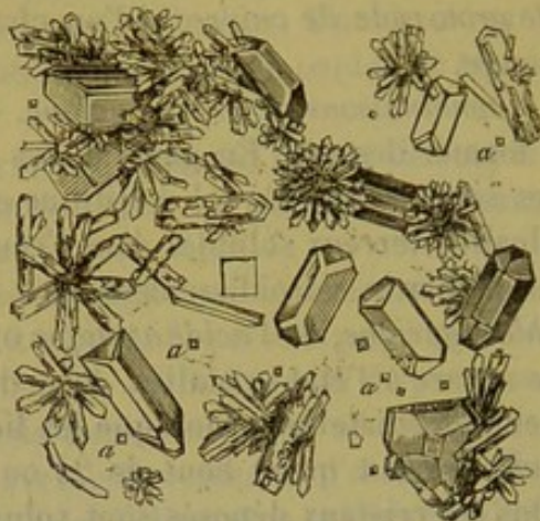
Fig. 57. — Urate de soude en cristaux groupés en étoiles, avec phosphate ammoniaco-magnésien et octaèdres d'oxalate de chaux (a) (sédiment d'une urine en fermentation alcaline avancée.)
