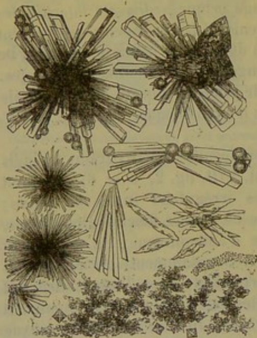
Fig. 92. — Urate de soude amorphe et cristallisé avec octaédres d'oxalate de chaux et coagulum muqueux (sédiment d'une urine en fermentation alcaline).
