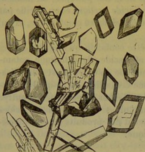
Fig. 65. — Glycocolle.
