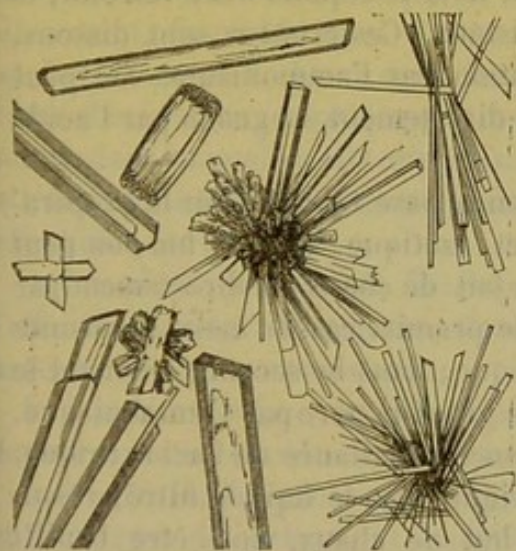
Fig. 75. — Chlorhydrate de guanine.
