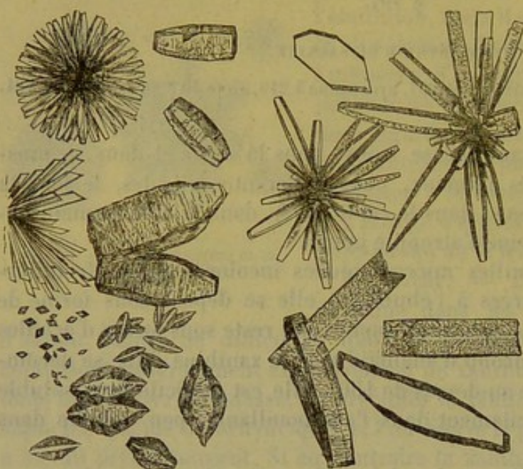
Fig. 72. — Azotate d'hypoxanthine. — Chlorhydrate d'hypoxanthine.
