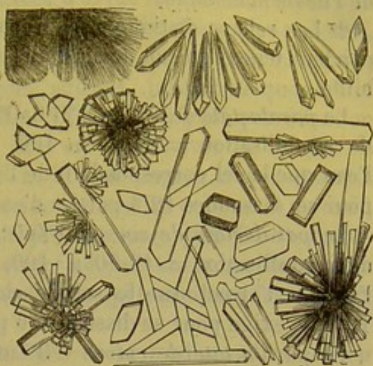
Fig. 55. — Lactate de zinc.
