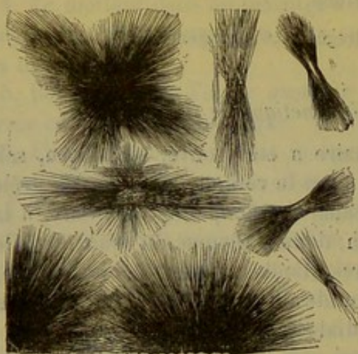
Fig. 52. — Lactate de chaux.
