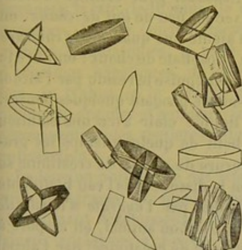
Fig. 79. — Créatinine.
