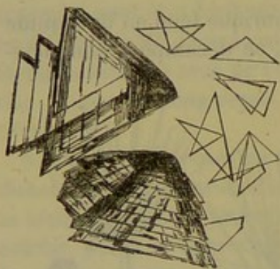
Fig. 63. — Kynurate de baryte.
