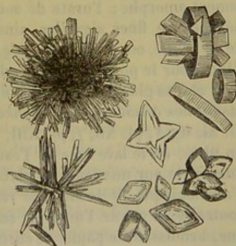
Fig. 60. — Acide urique (sédiment).
