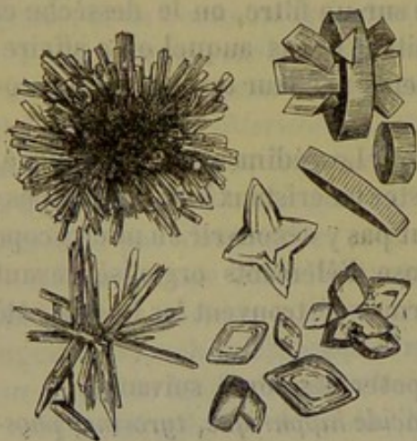
Fig. 86. — Acide urique (sédiment).
