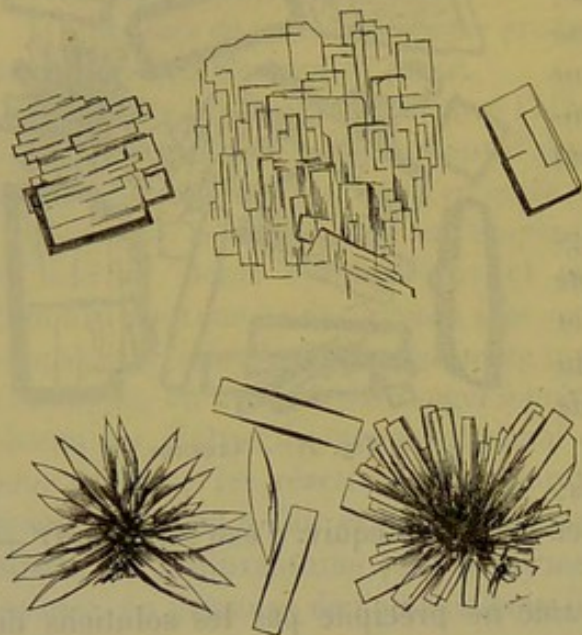
Fig. 78. — Sarkosine pure. et sulfate de sarkosine.
