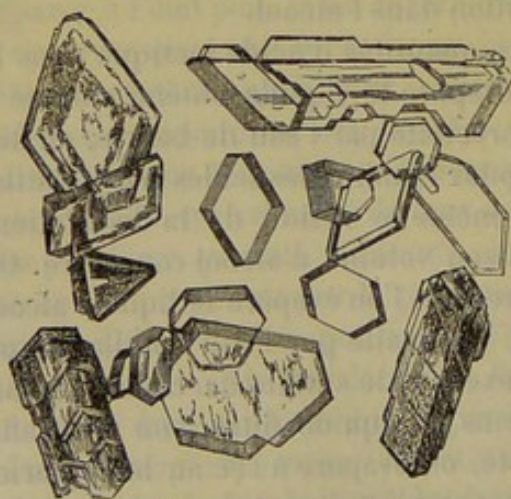
Fig. 54. — Acide succinique.
