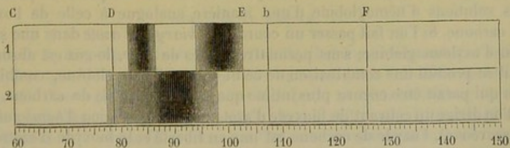
Fig. 45. — Spectres de l'hémoglobine.
