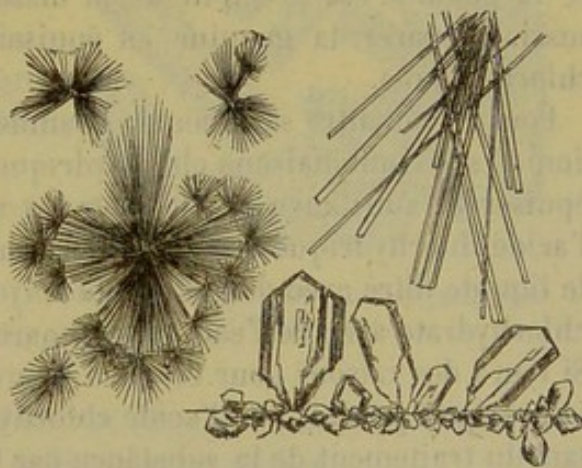
Fig. 74. — Azotate de guanine.
