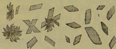
Fig. 45. Cristaux d'hémine.
