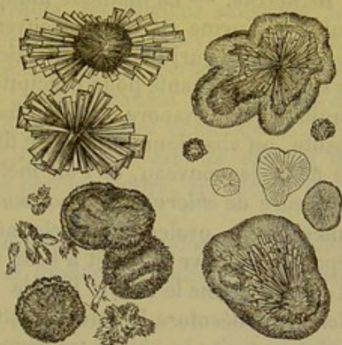
Fig. 80. — Chlorure de zinc et de créatinine
