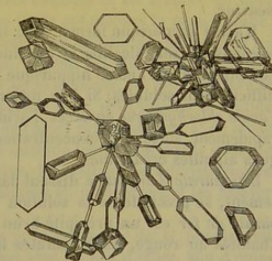
Fig. 64. — Acide hippurique.
