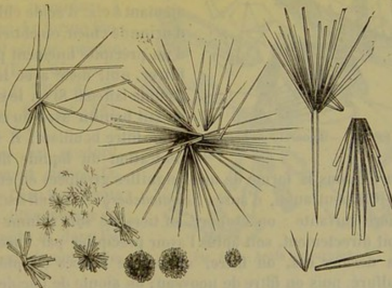
Fig. 62 — Acide kynurique.
