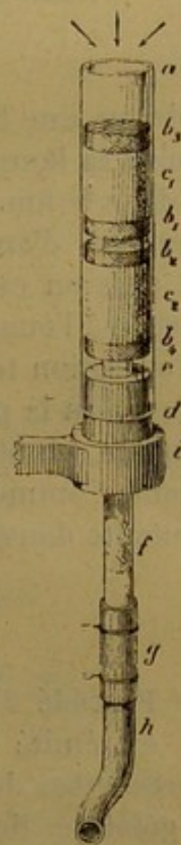
Fig. 219. — Filtre à sable de Petri pour les germes de l'air.
