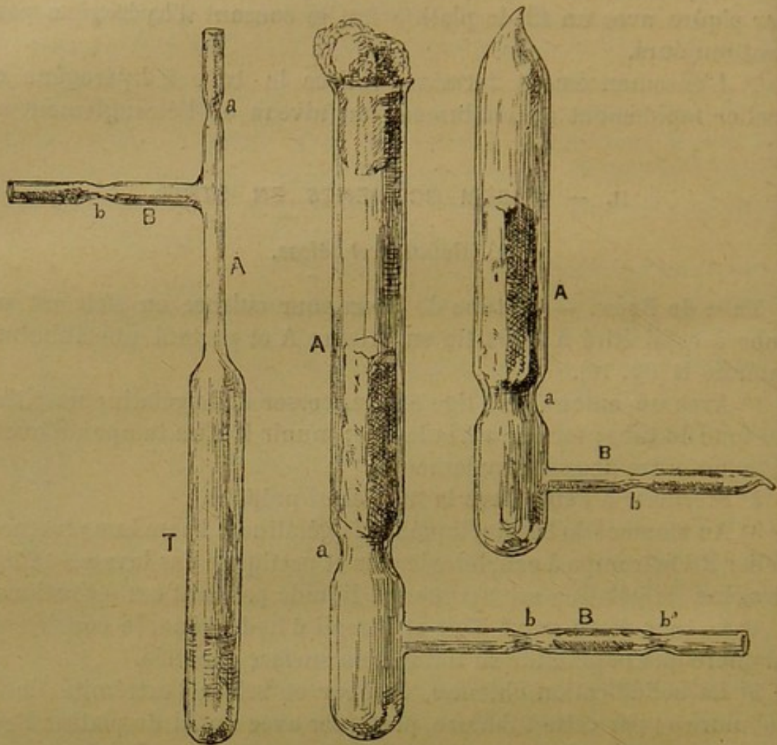
Fig. 76. — Tube de Roux pour ensemencement en strie.
