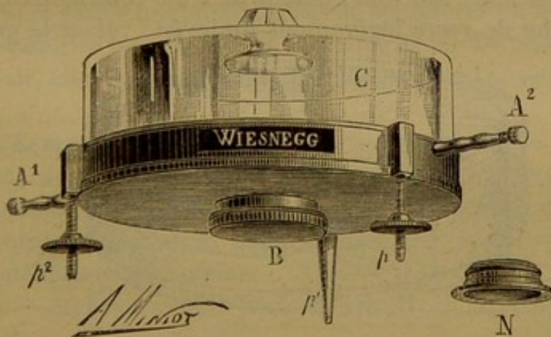
Fig. 60. — Appareil pour plaques de gélatine.
