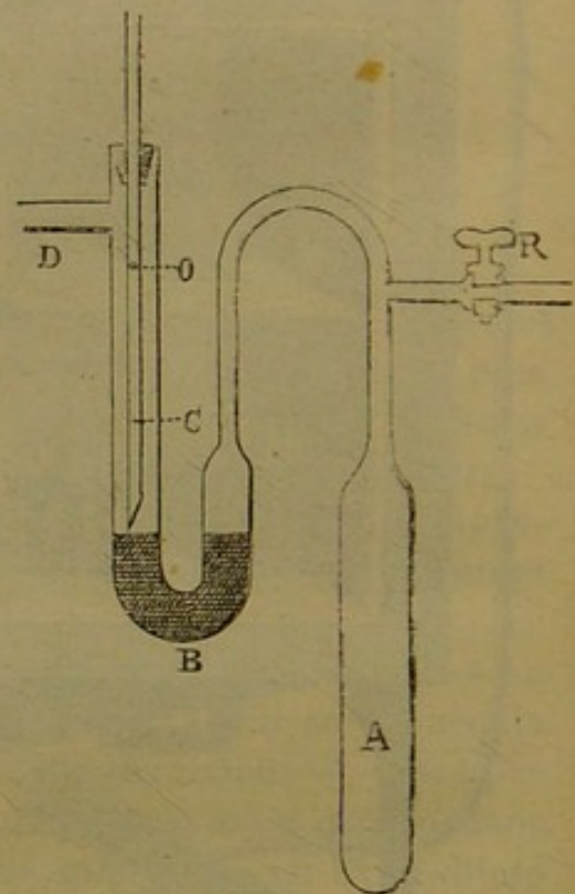
Fig. 51. — Régulateur de Bohr.
