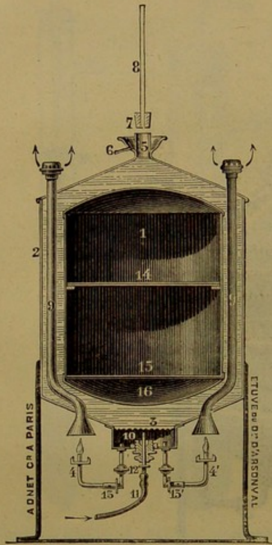
Fig. 53. — Coupe de l'étuve autorégulatrice de d'Arsonval.
