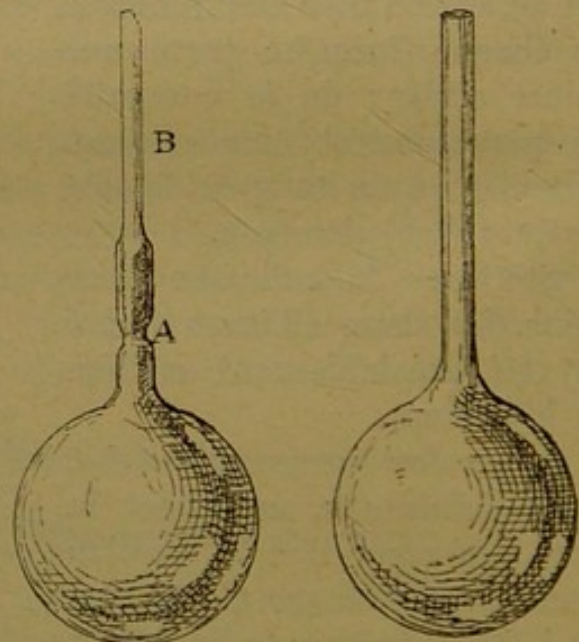
Fig. 71. — Disposition pour la culture des anaérobies dans les ballons à long col.
