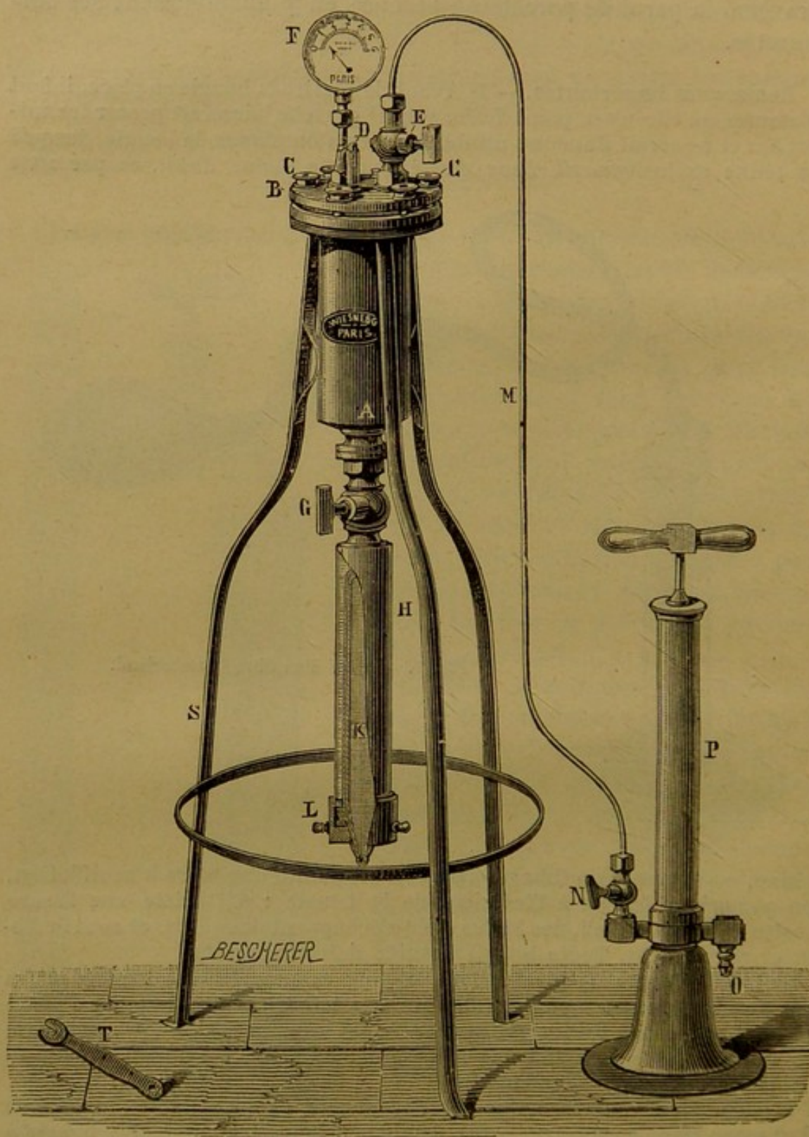
Fig. 10. — Filtre à pression graduée.
