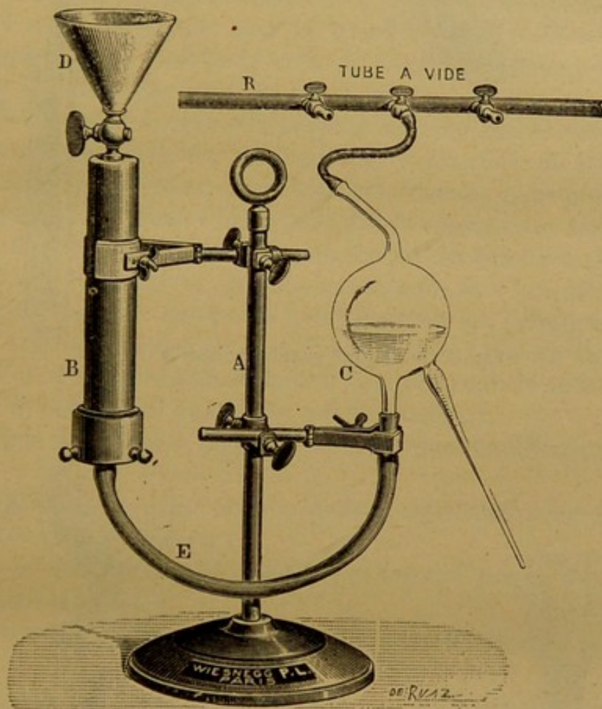
Fig. 16. — Appareil à filtration de L. Martin.
