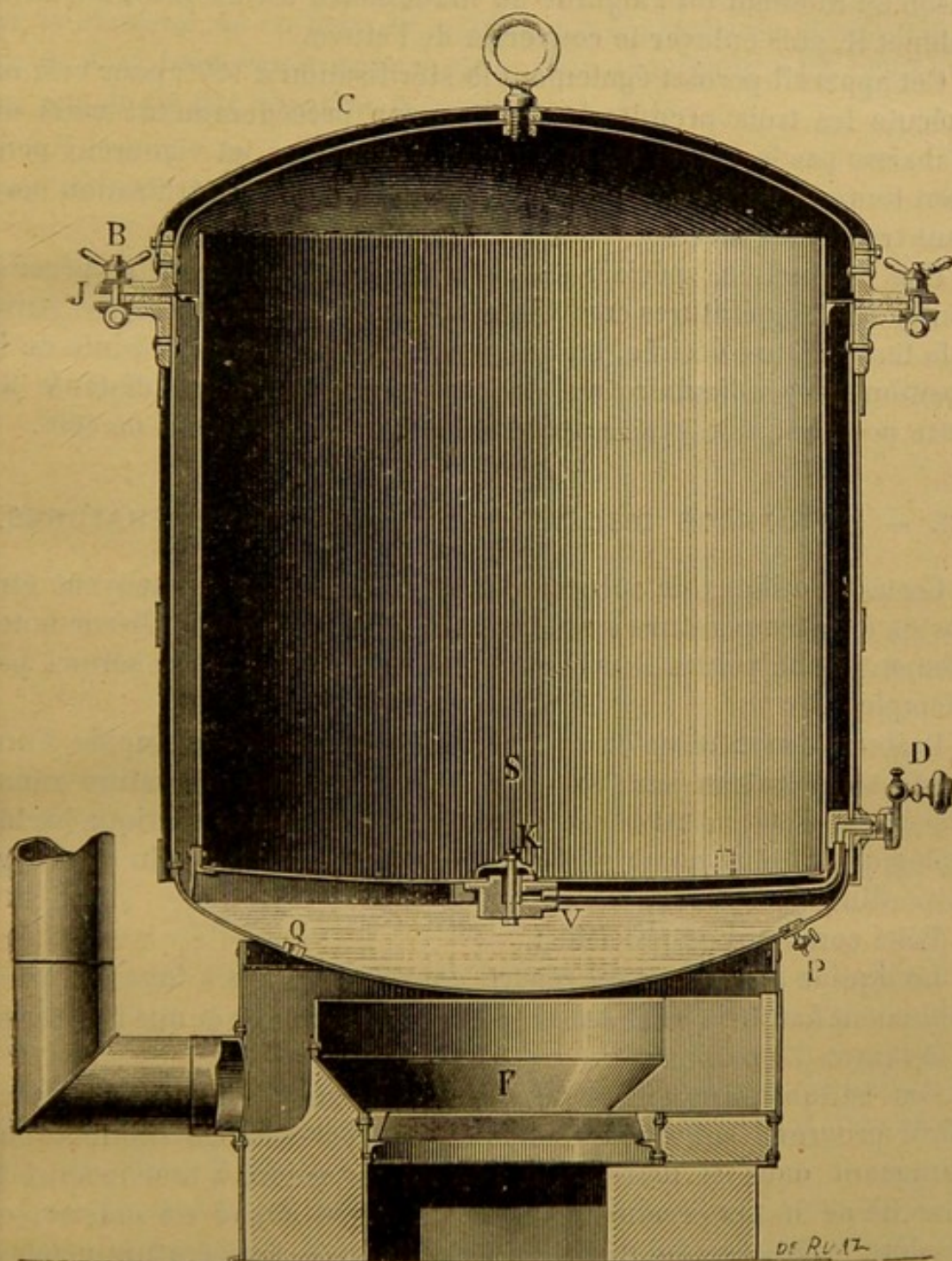
Fig. 6. — Appareil à stérilisation de Vaillard et Besson.
