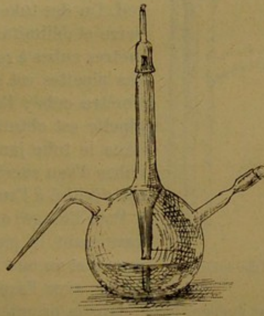
Fig. 222. — Ballon de Miquel.
