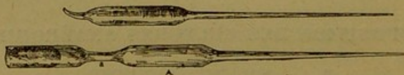
Fig. 68. — Préparation de la pipette de Roux.
