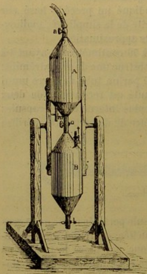
Fig. 218. — Aspirateur à eau.
