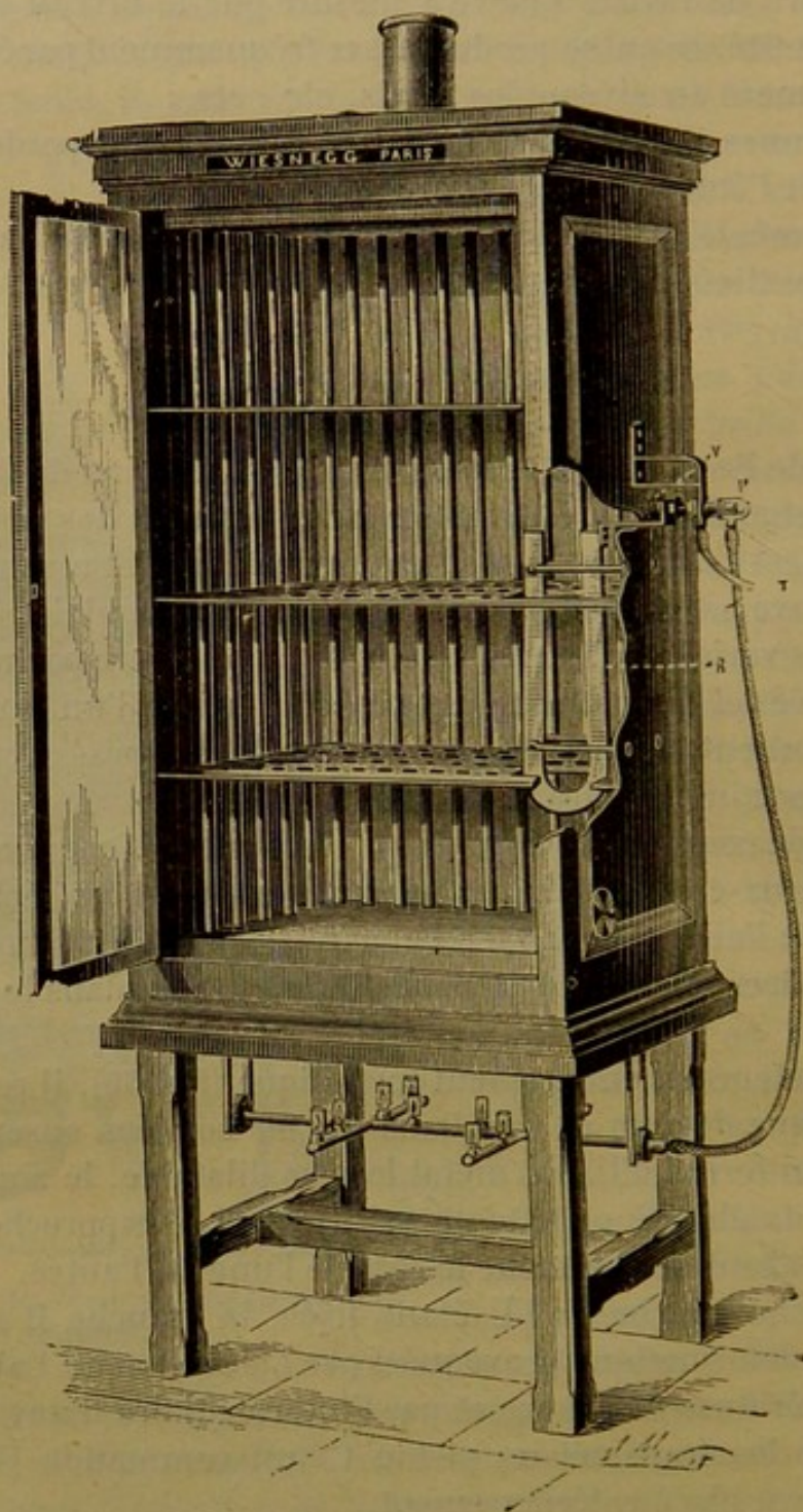
Fig. 54. — Étuve de Pasteur modifiée par Roux.
