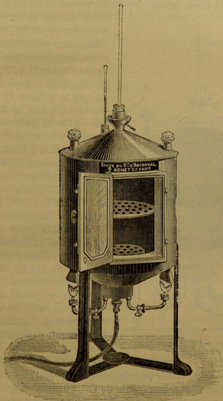
Fig. 52. — Nouvelle étuve autorégulatrice de d'Arsonval.
