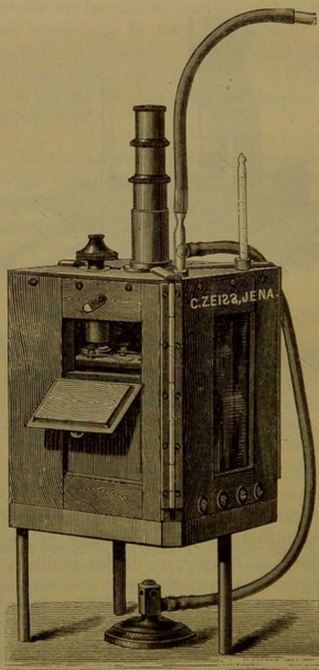
Fig. 90. — Étuve de Zeiss pour observations au microscope.
