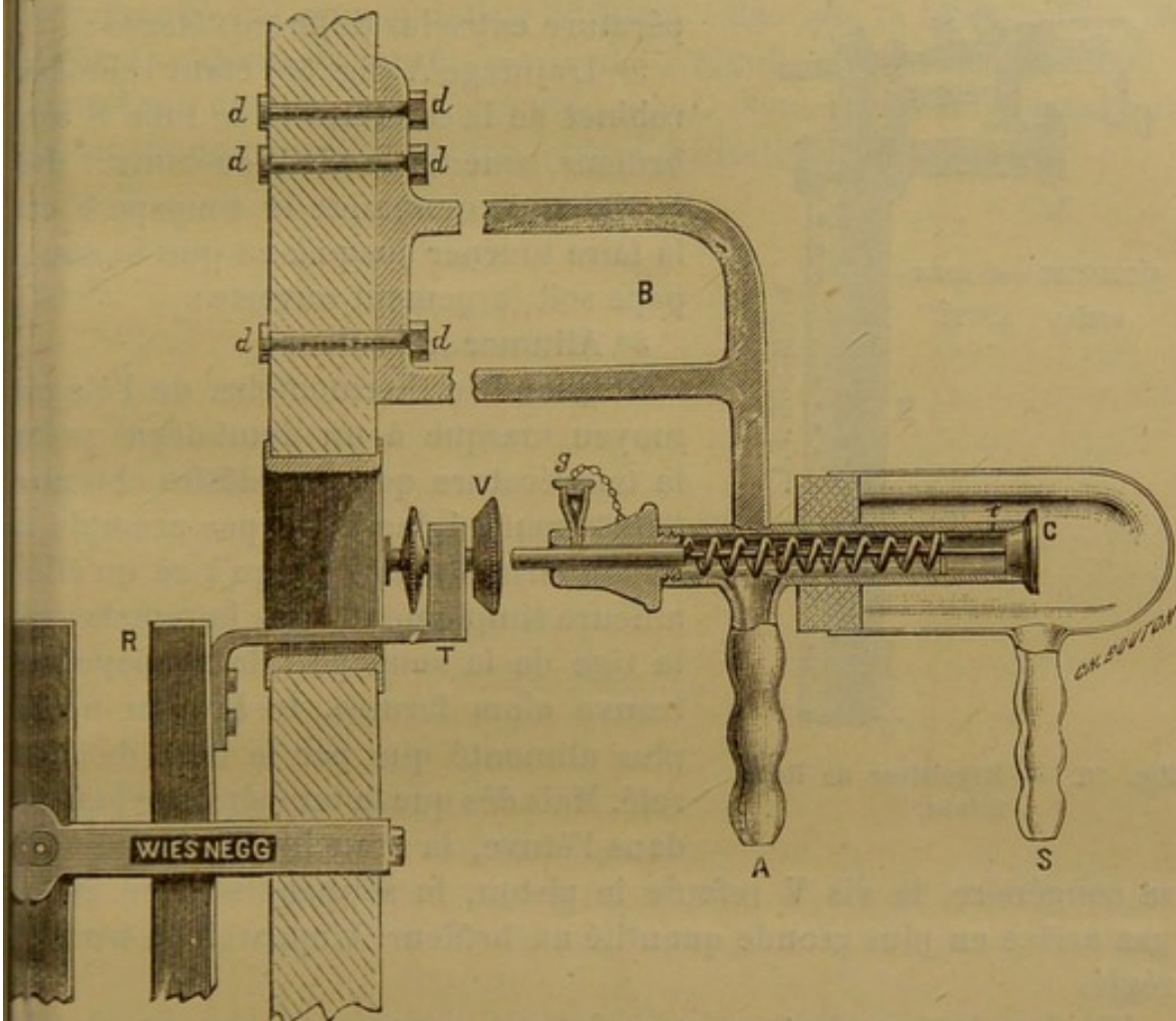
Fig. 55. — Régulateur métallique de Roux.
