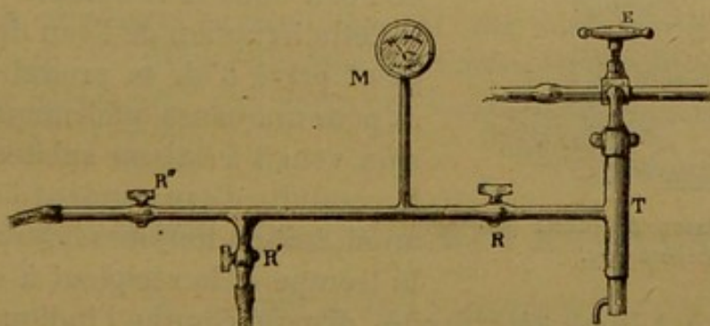
Fig. 65. — Disposition d'une trompe à eau.
