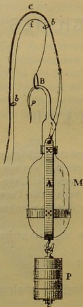
Fig. 215. — Appareil pour prélever les eaux à diverses profondeurs.
