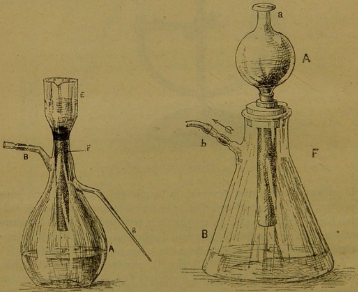
Fig. 19. — Filtre de Kitasato.
