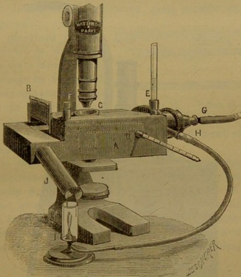
Fig. 87. — Chambre chaude de Vignal.
