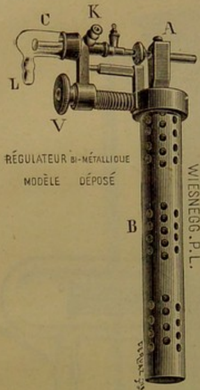
Fig. 56. — Régulateur de Roux à tube.
