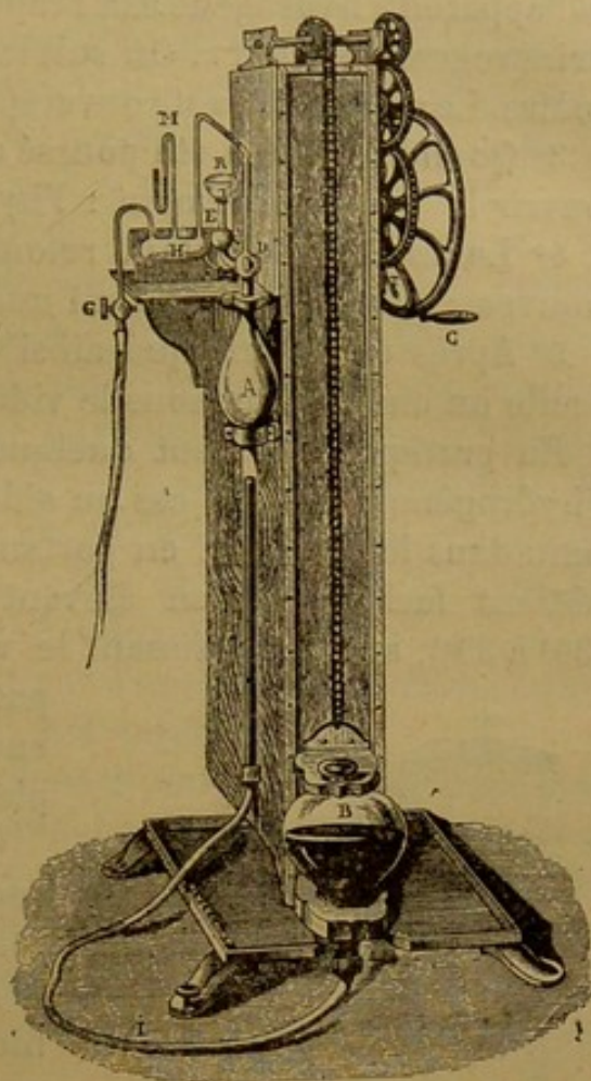
Fig. 64. — Pompe à mercure.
