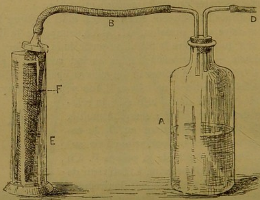
Fig. 12. — Appareil pour filtrer dans le vide.
