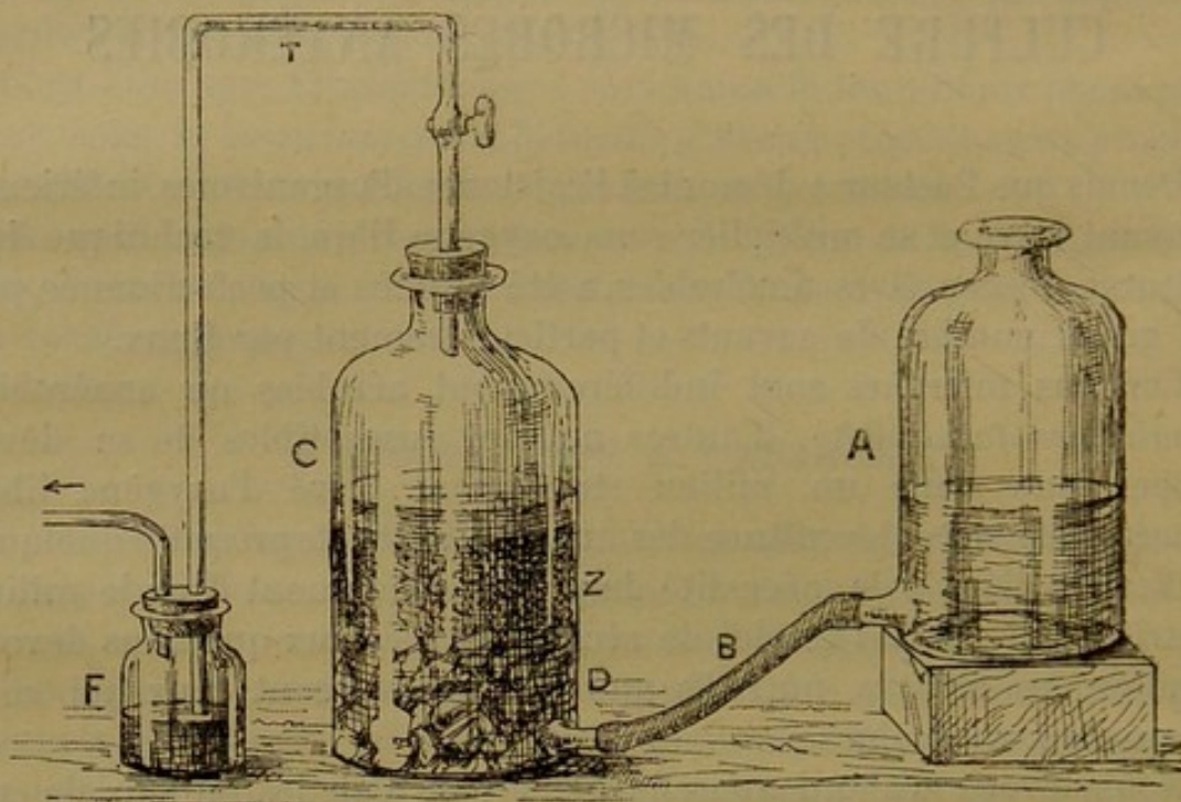
Fig. 63. — Appareil à dégagement continu d'hydrogène.
