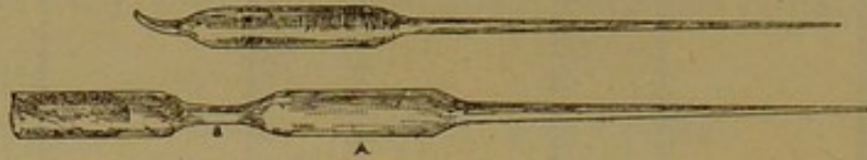
Fig. 47. — Préparation des ampoules pour la conservation des cultures à l'abri de l'air.
