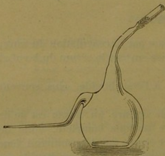
Fig. 25. — Matras répartiteur.
