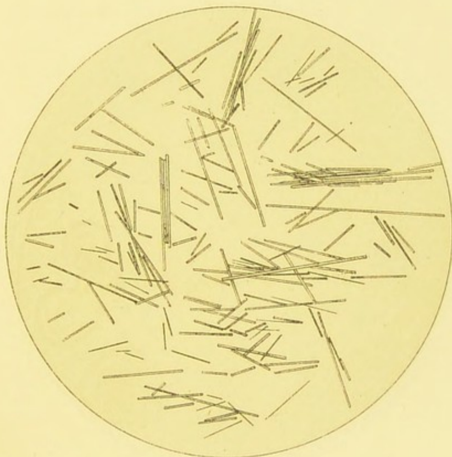
FIG. 83.—Tyrosin.
