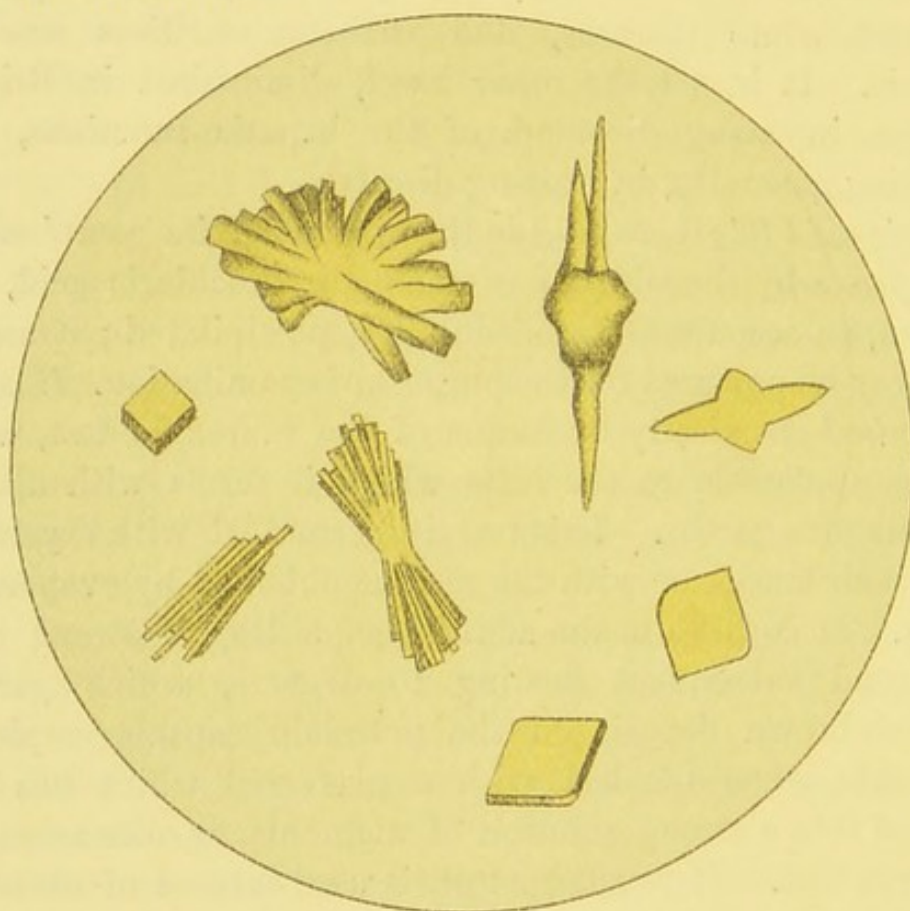
FIG. 73.—Uric acid.
