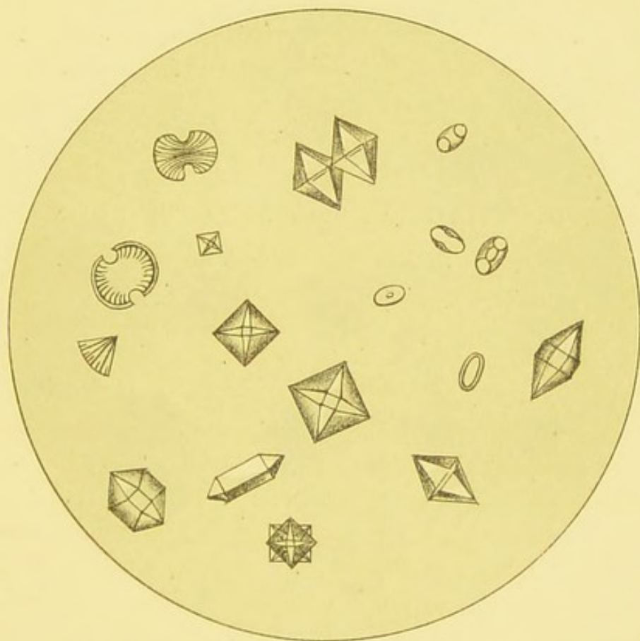
FIG. 81.—Calcium oxalate.
