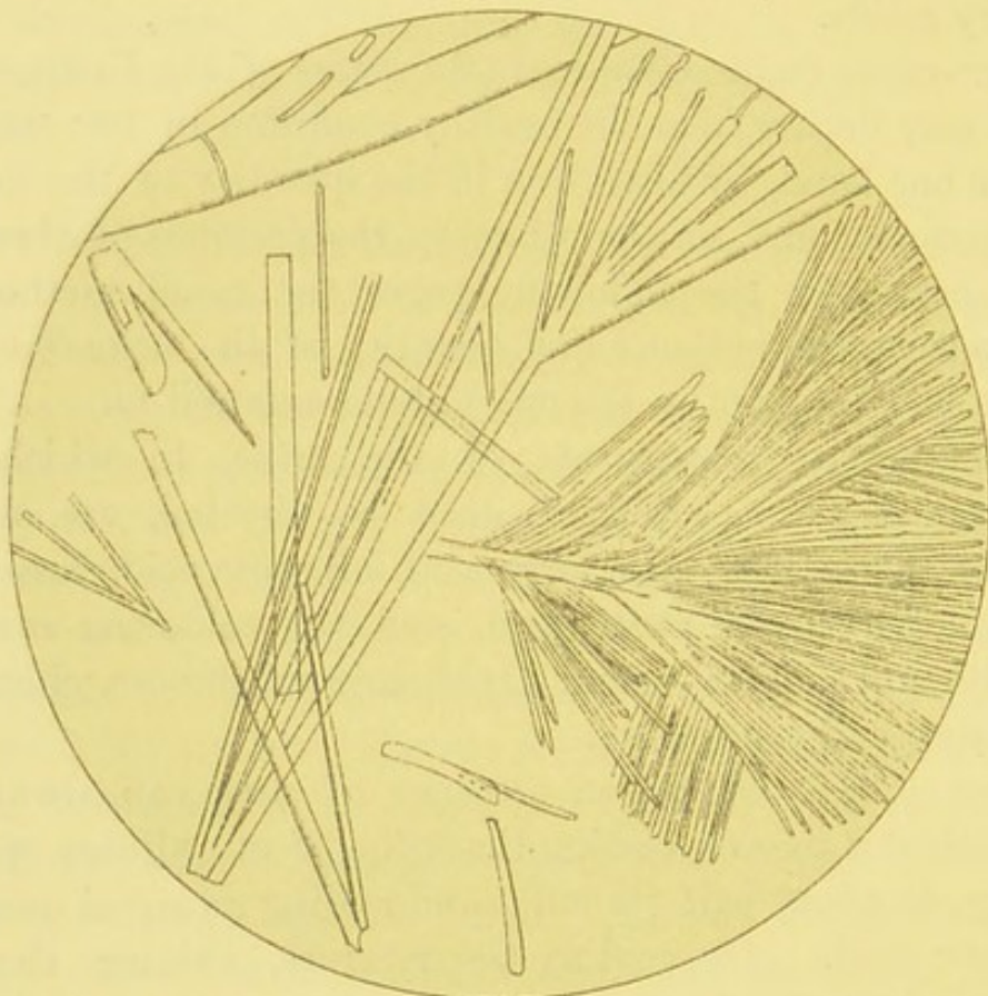
FIG. 70.—Urea.
