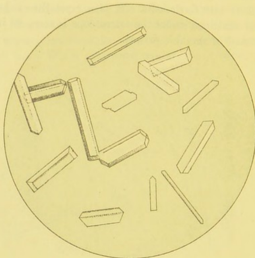
FIG. 78.—Kreatinin.
