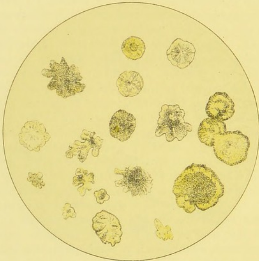
FIG. 82.—Leucin.
