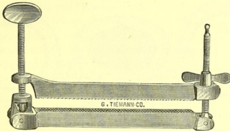
FIG. 41.—T. S. WELLS'S CLAMP.
