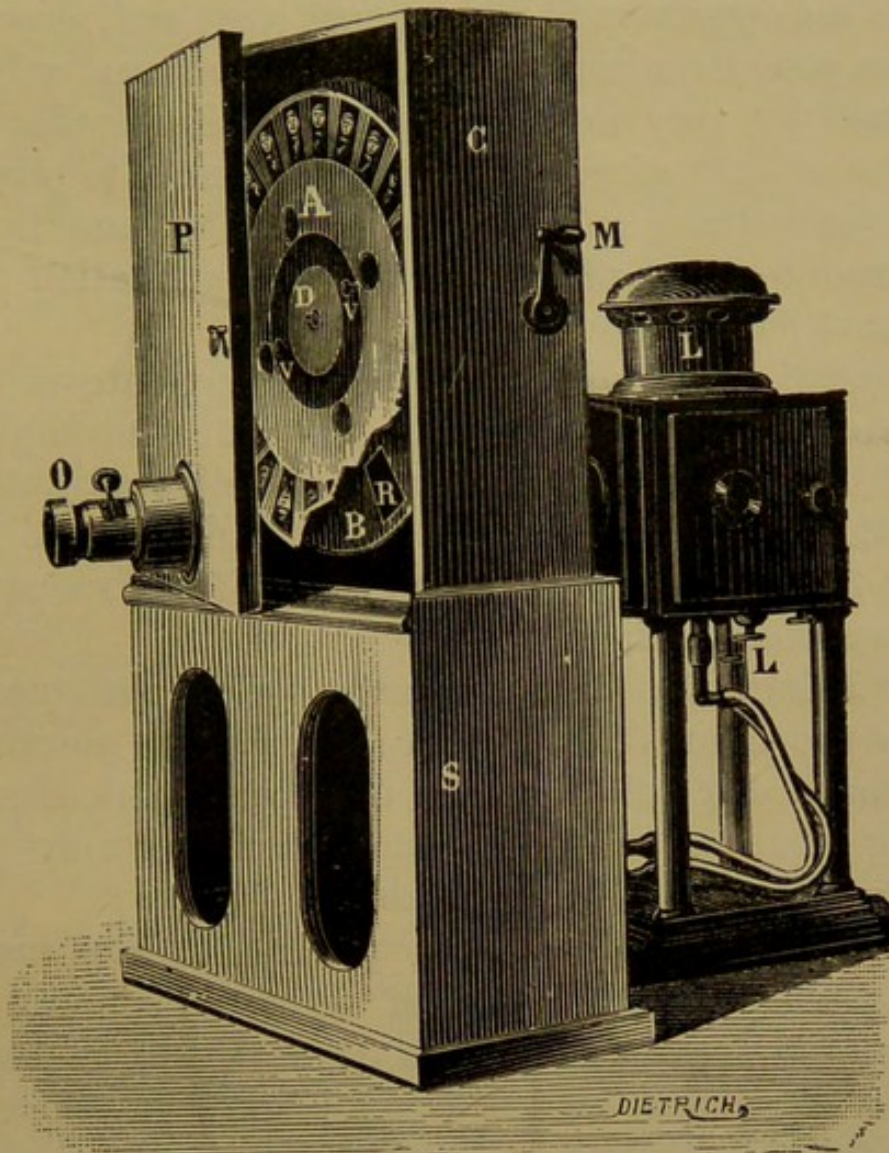
FIG. 204.—Demeny's photophone.
