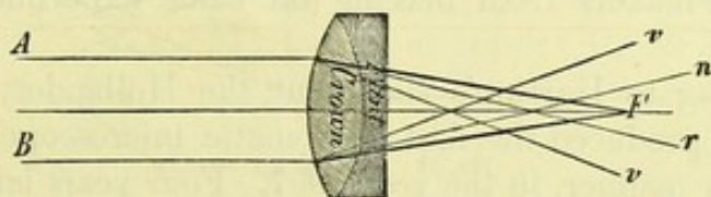
Fig. 14. Achromatic lens.
