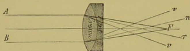
FIG. 14. Achromatic lens.
