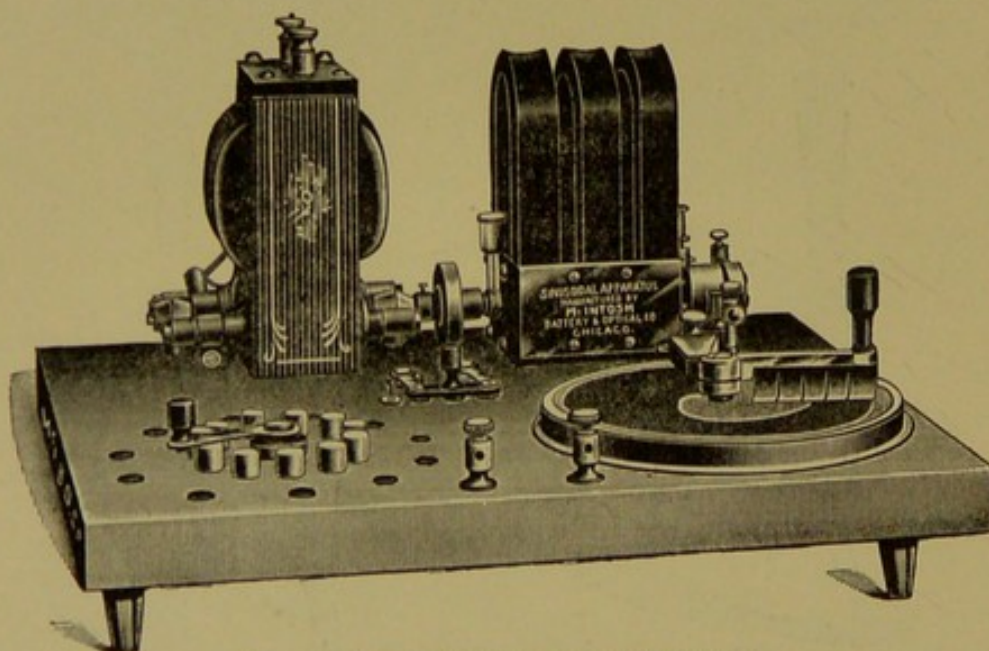
FIG. 73.—Sinusoidal Apparatus (McIntosh).
