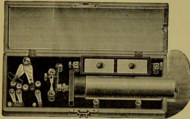
FIG. 58.—Pocket Apparatus (Kidder).
