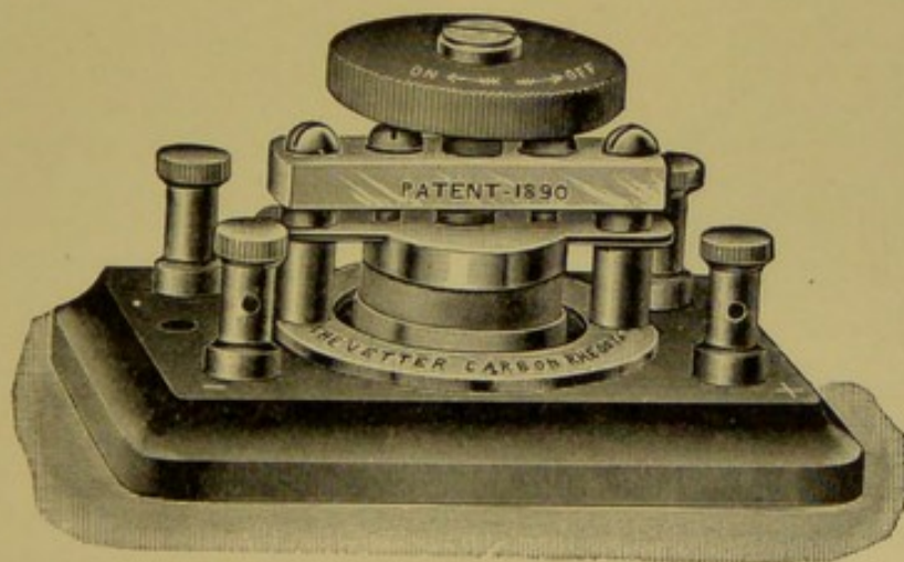
FIG. 75.—The Carbon Rheostat (Vetter).
