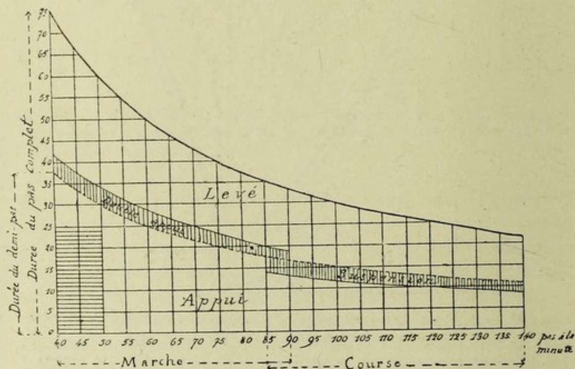
Fig. 364. — Comparaison de la durée de l'appui et du lever du pied, du double appui et de la suspension dans la marche et la course (DEMENY).
