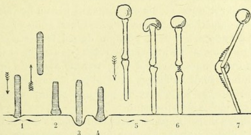
Fig. 439. — Différents cas qui se présentent dans la chute d'un corps suivant l'élasticité de ce corps et celle du sol.
