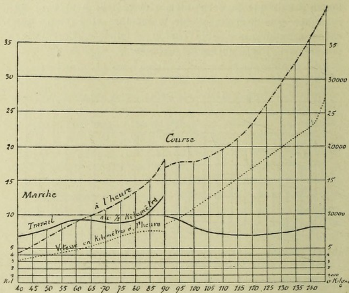
Fig. 542. — Comparaison du travail à l'heure et au kilomètre dans des allures dont la cadence s'accélère régulièrement ; variations correspondantes de la vitesse.
