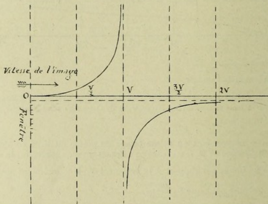
Fig. 534. — Loi du flou de l'image photographique obtenue avec un obturateur à fente étroite se mouvant dans le même sens que le point lumineux à photographier.
