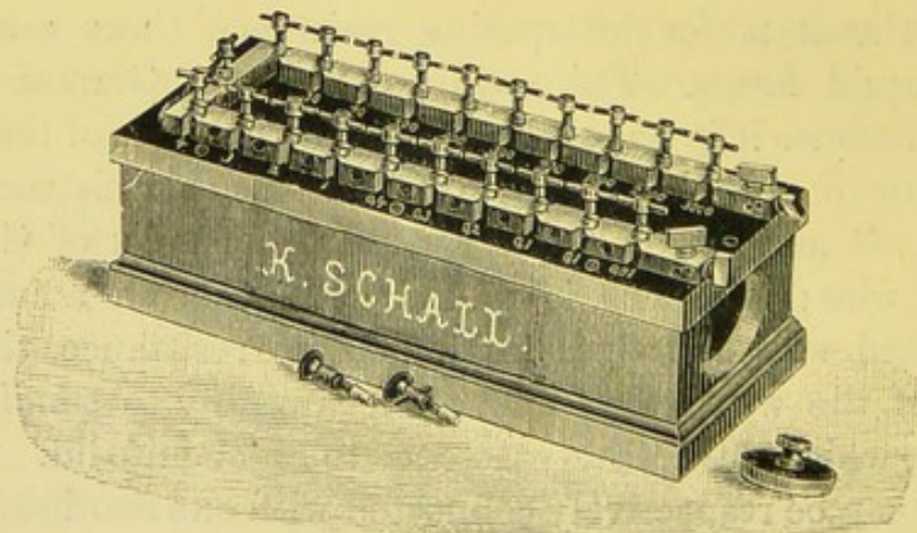
FIG. 54.—PLUG RHEOSTAT.
