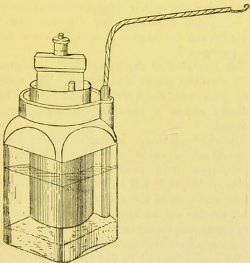
FIG. 14.—LECLANCHÉ CELL.
