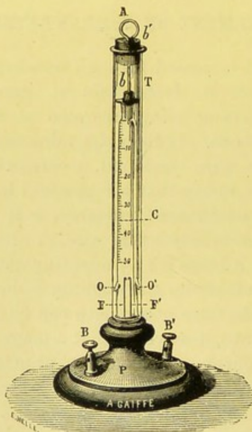
FIG. 35.—VOLTAMETER.
