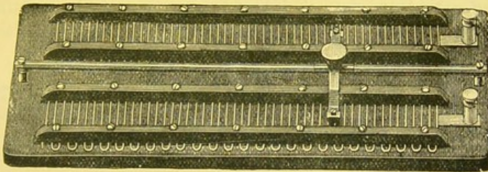
FIG. 55.—SIMPLE RHEOSTAT.
