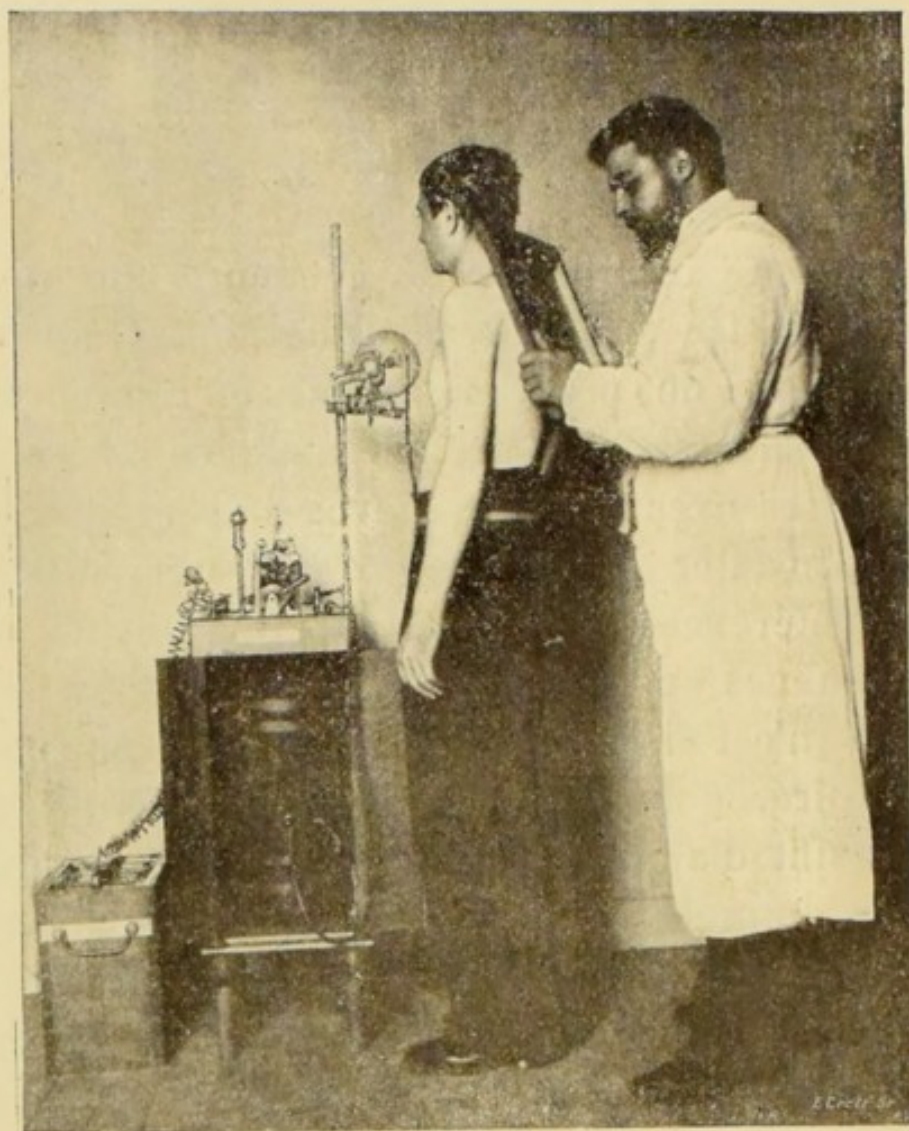
Fig. 1. — Un examen radioscopique du thorax à l'hôpital Tenon. A. Accumulateurs (batterie de trois). — B. Transformateur et interrupteur de MM. Wydts et Rochefort. — C. Ampoule à vide. — D. Écran fluorescent.
