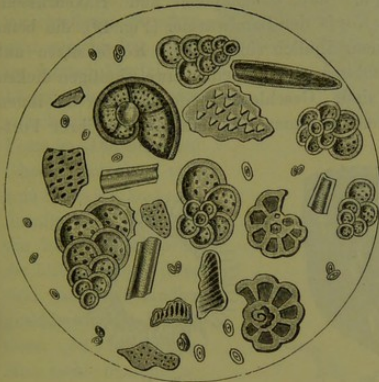
Fig. 38. Schreibkreide nach Zittel.
