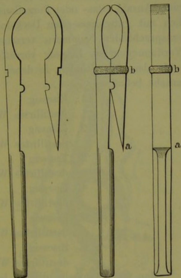
Fig. 17. Halter für Kochgläschen. \frac{1}{2} nat. Grösse.
