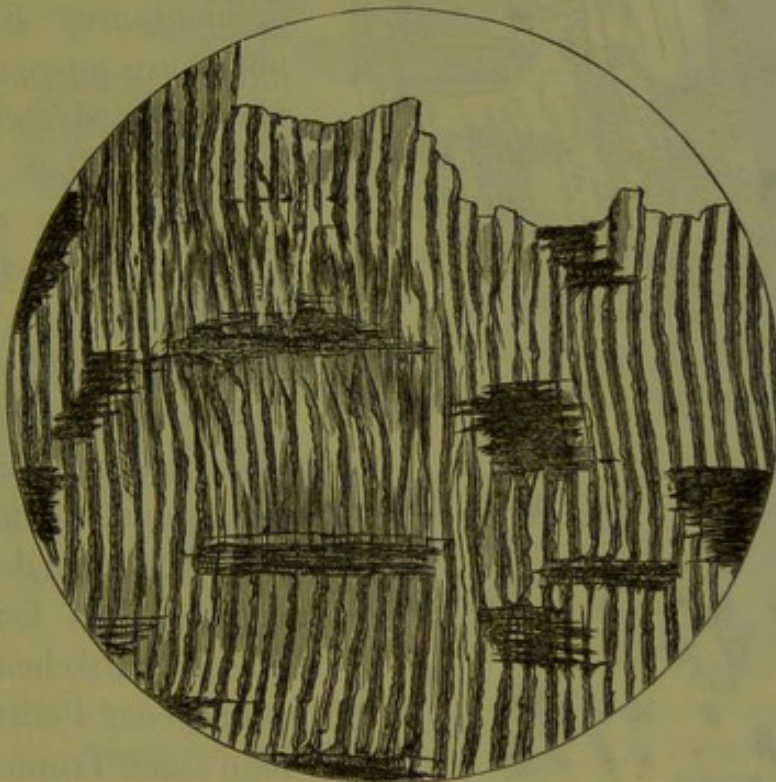
Fig. 35. Steinkohle. Dünnschliff.
