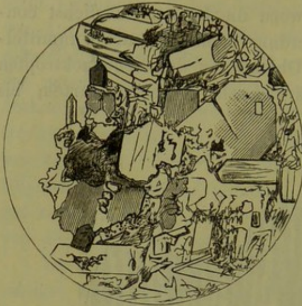
Fig. 36. Lava vom Vesuv. Dünnschliff.
