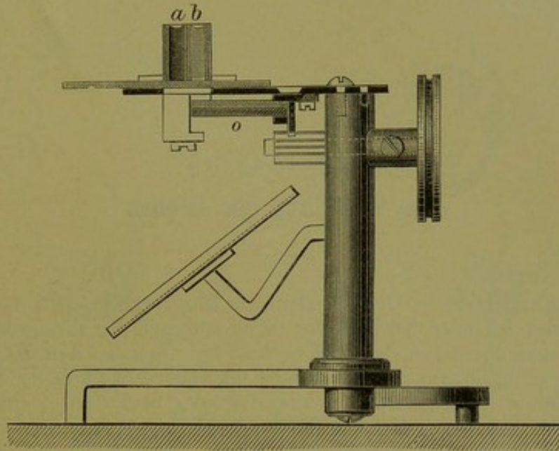
Fig. 5. Hämometer von v. Fleischl: a , b das Nöpfchen; o die keilförmige, rothe Glasplatte, senkrecht gegen die Ebene der Figur verschiebbar.
