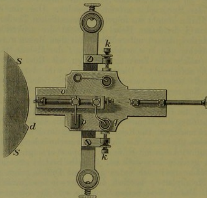
und Fig. 75 B. Myographion von Helmholtz.
