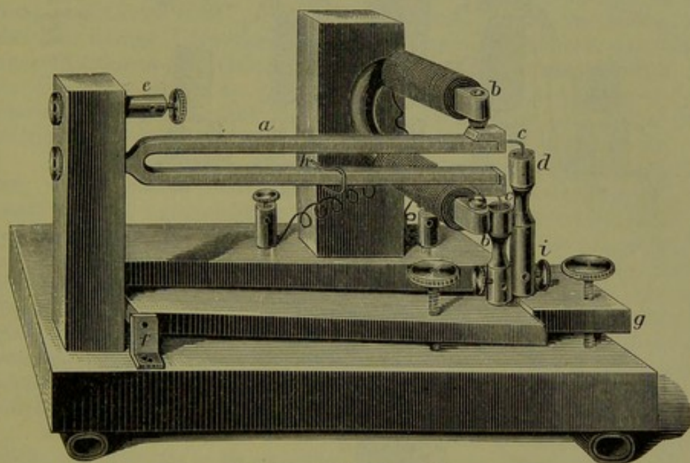
Fig. 233. Unterbrechergabel.
