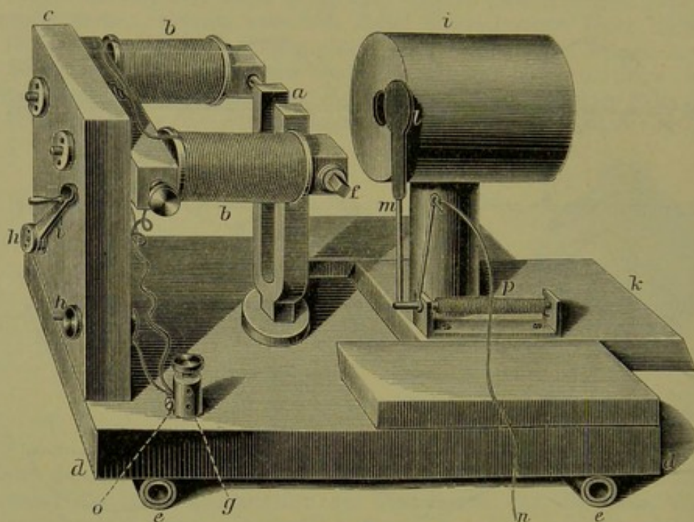
Fig. 232. Elektromagnetische Stimmgabel mit Resonator.
