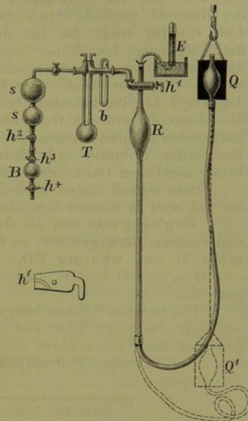
Fig. 50. Quecksilberluftpumpe zur Blutentgasung nach Pflüger.
