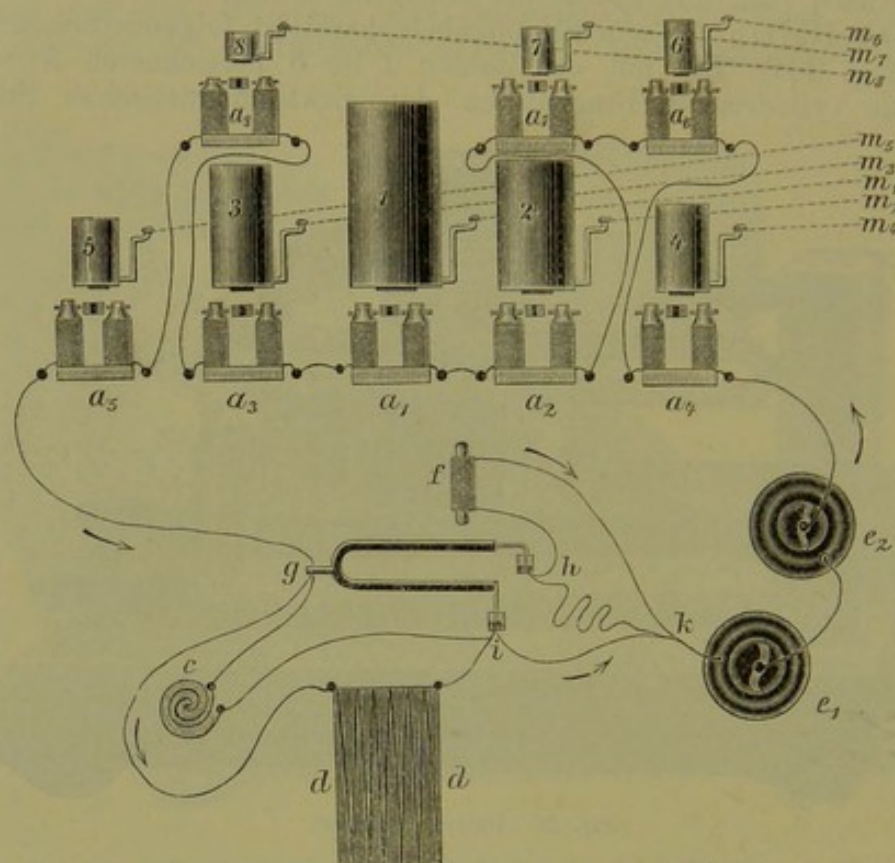
Fig. 234. Stimmgabelapparat von Helmholtz.
