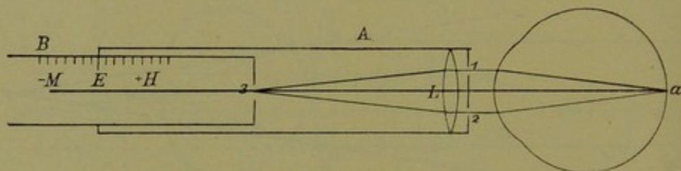
Fig. 171. Optometer.
