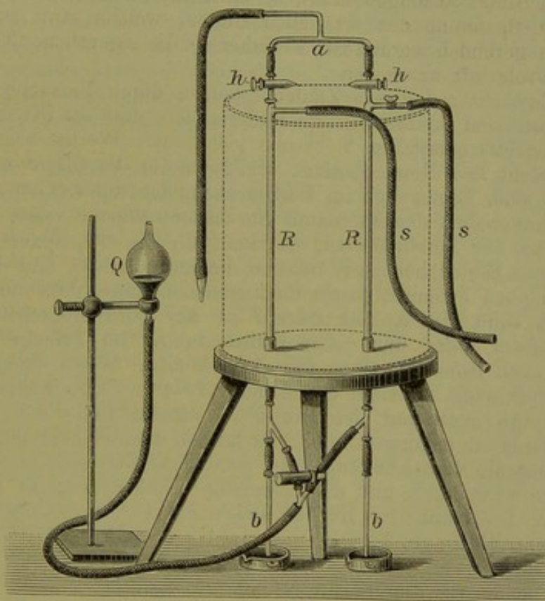
Fig. 52. Aërotonometer von Pflüger.
