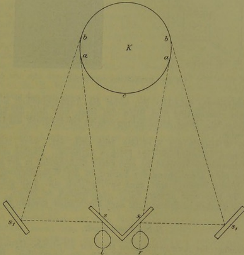
Fig. 213. Telestereoskop von Helmholtz.
