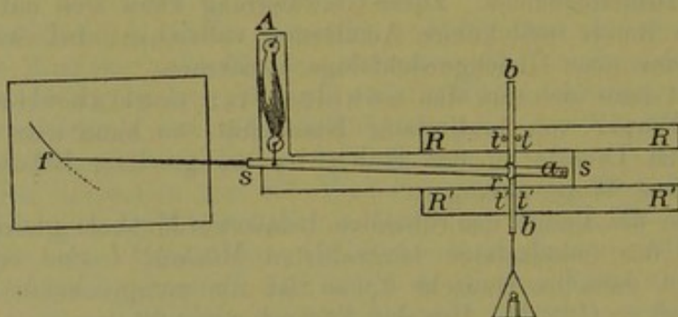
Fig. 72. Myographion von Blix.
