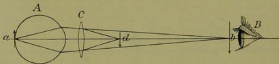
Fig. 181. Entwerfung eines reellen Bildes der Netzhaut.
