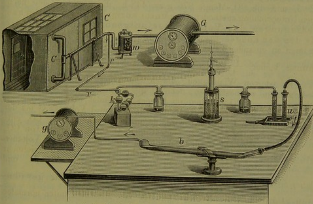
Fig. 54. Respirationsapparat von Pettenkofer.
