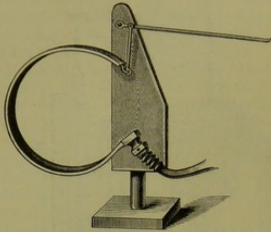
Fig. 23. Federmanometer von Fick.
