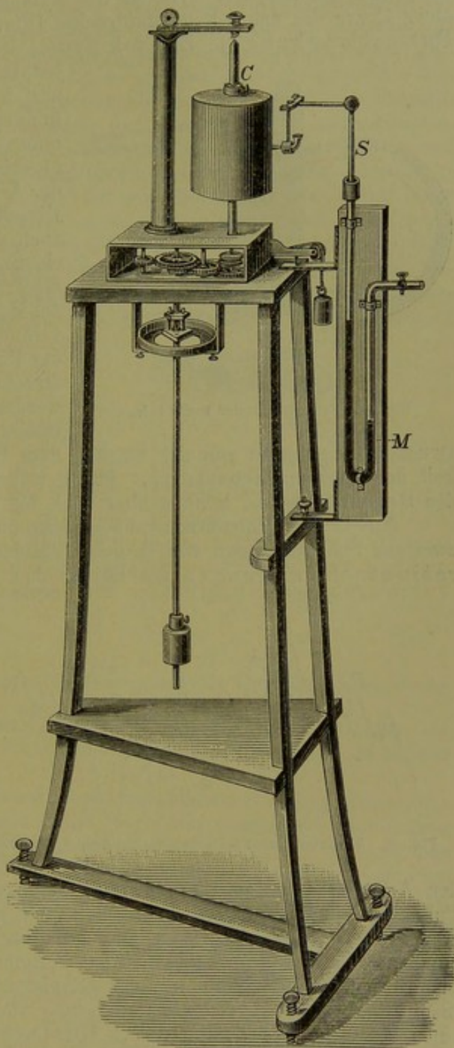
Fig. 22. Kymographion mit Quecksilbermanometer nach Ludwig.
