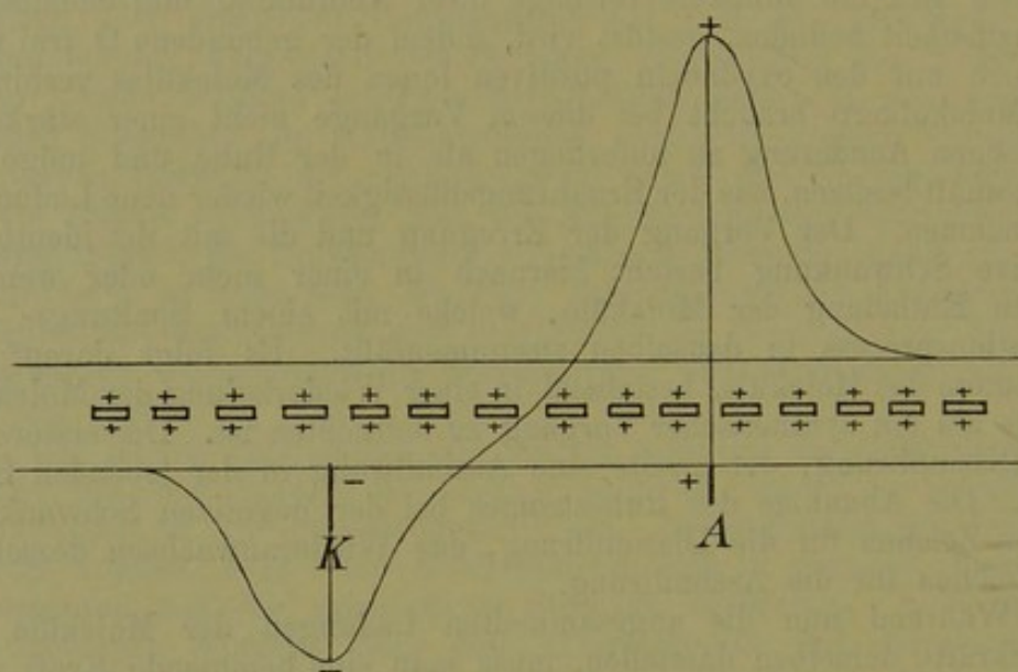
Fig. 127. Polarisation einer Molekülreihe.
