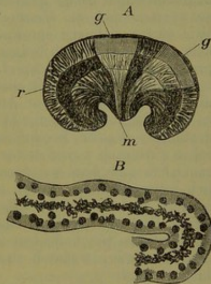
Fig. 62. A Niere mit indigschwefelsaurem Natron injicirt, nach Heidenhain: r Rinde, m Mark, g geätzte Partien; B ein gewundenes Harncanälchen.
