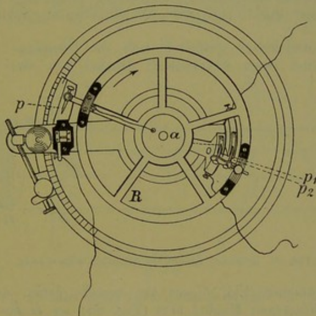
Fig. 86 B. Differentialrheotom von Bernstein.
