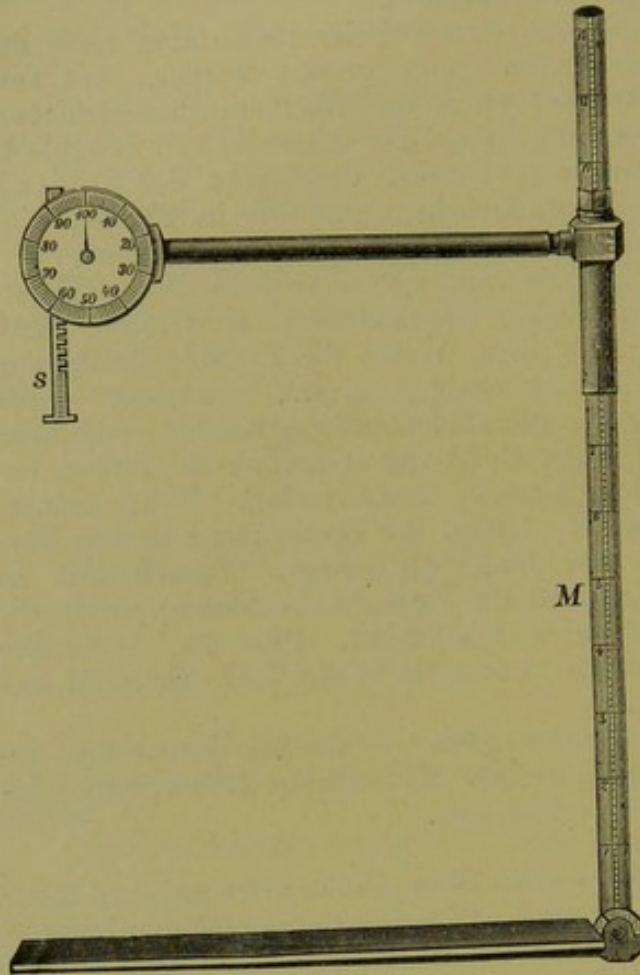
Fig. 41. Thoracometer von Sibson.
