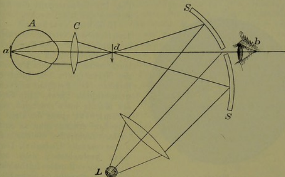
Fig. 182 A. Augenspiegel nach Ruete.
