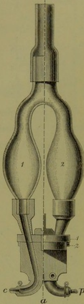
Fig. 29. Stromuhr von Ludwig.
