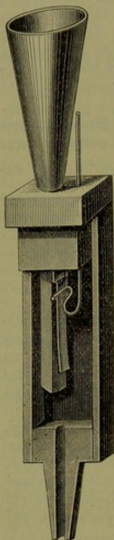
Fig. 102 A. Eine Zungenpfeife mit Ansatzrohr.
