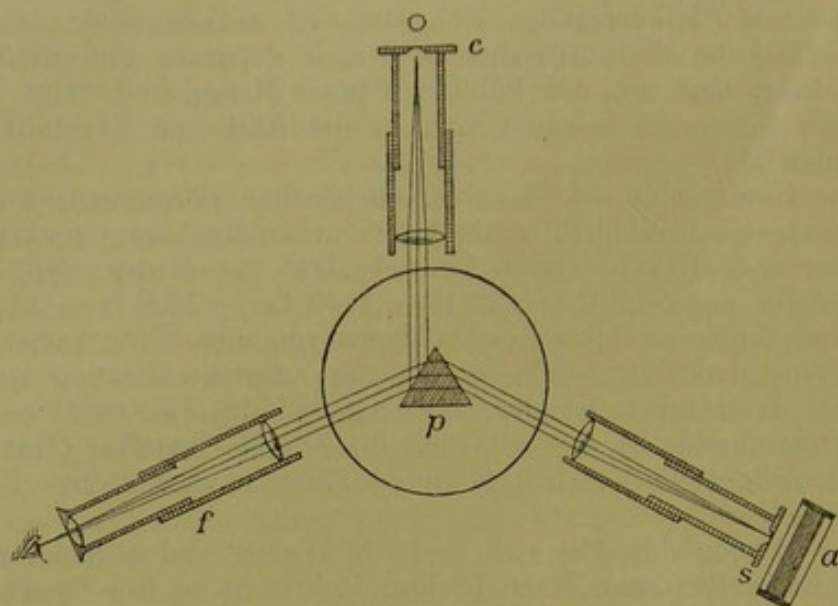
Fig. 3. Spektralapparat: p Prisma, s Spalt, c Scala, f Fernrohr, a Gefäß mit Blutlösung.
