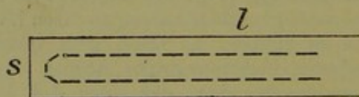
Fig. 91. Parelektronomie.
