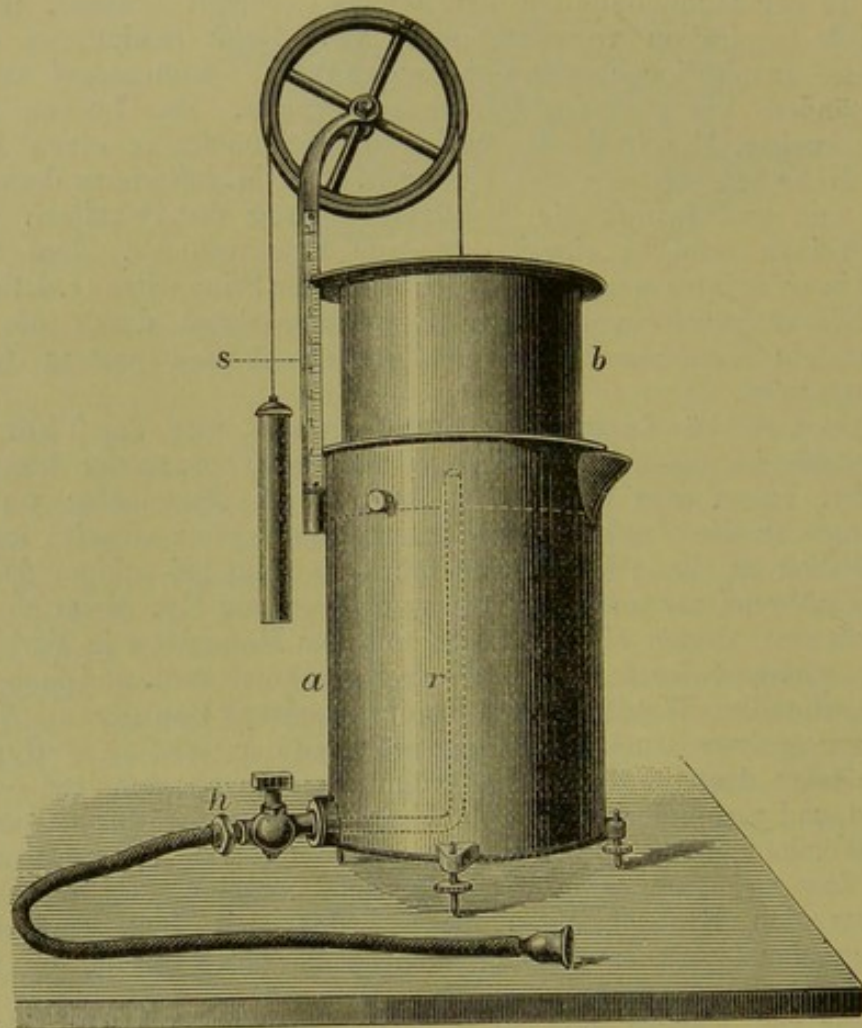
Fig. 45. Spirometer von Hutchinson.
