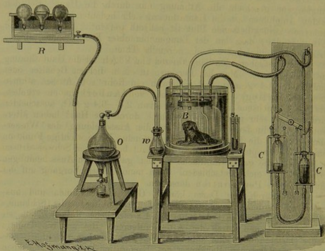
Fig. 53. Respirationsapparat von Regnault und Reiset.
