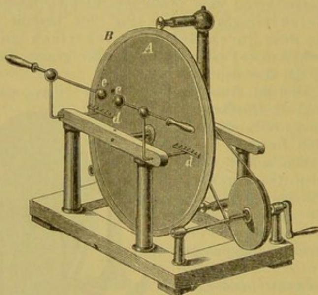
Holtz'sche Influenzmaschine von der Seite der beweglichen Scheibe A aus.
