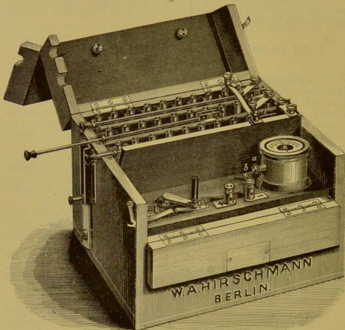
Leicht transportabler Apparat für constanten Strom mit 30 Elementen, Galvanometer, Stromwender und Elementenzähler.
