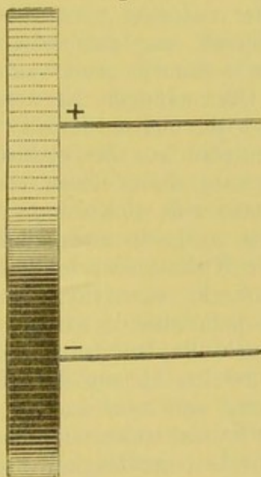
Schema des Eckhard-Pflüger'schen Elektrotonus an Nerven. Die Stärke der Schattirung zeigt den Grad der Erregbarkeitszu- und -abnahme.
