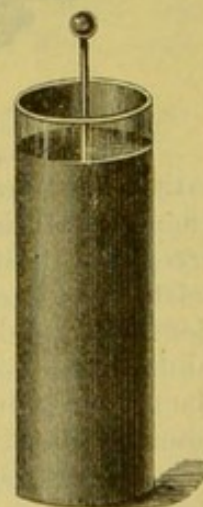
Kleist'sche Flasche.
