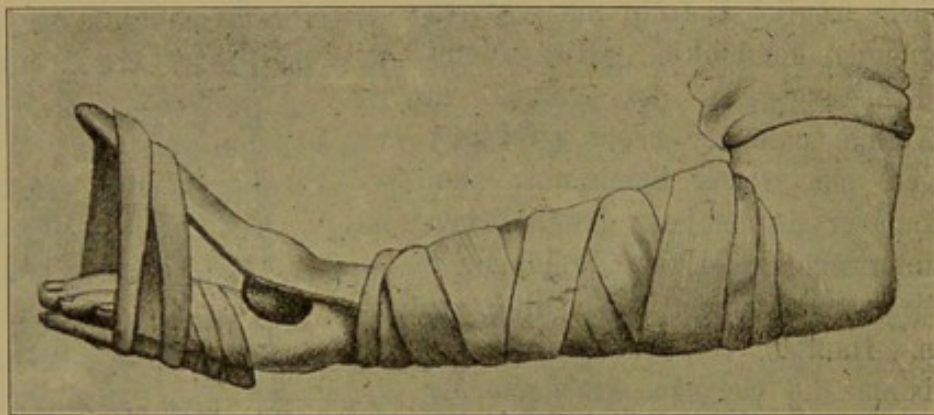
Verwendung der dorsalen Gipshanschiene zur Streckung von Kontrakturen des Handgelenkes mittelst Gummizuges.
