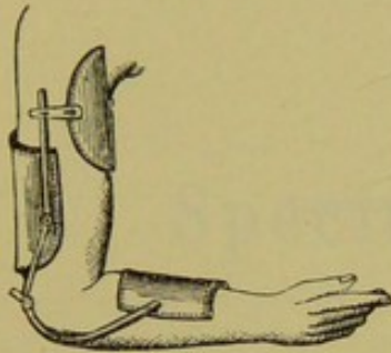
Apparat zur Streckung von Ellbogen-Kontrakturen nach Bidder.
