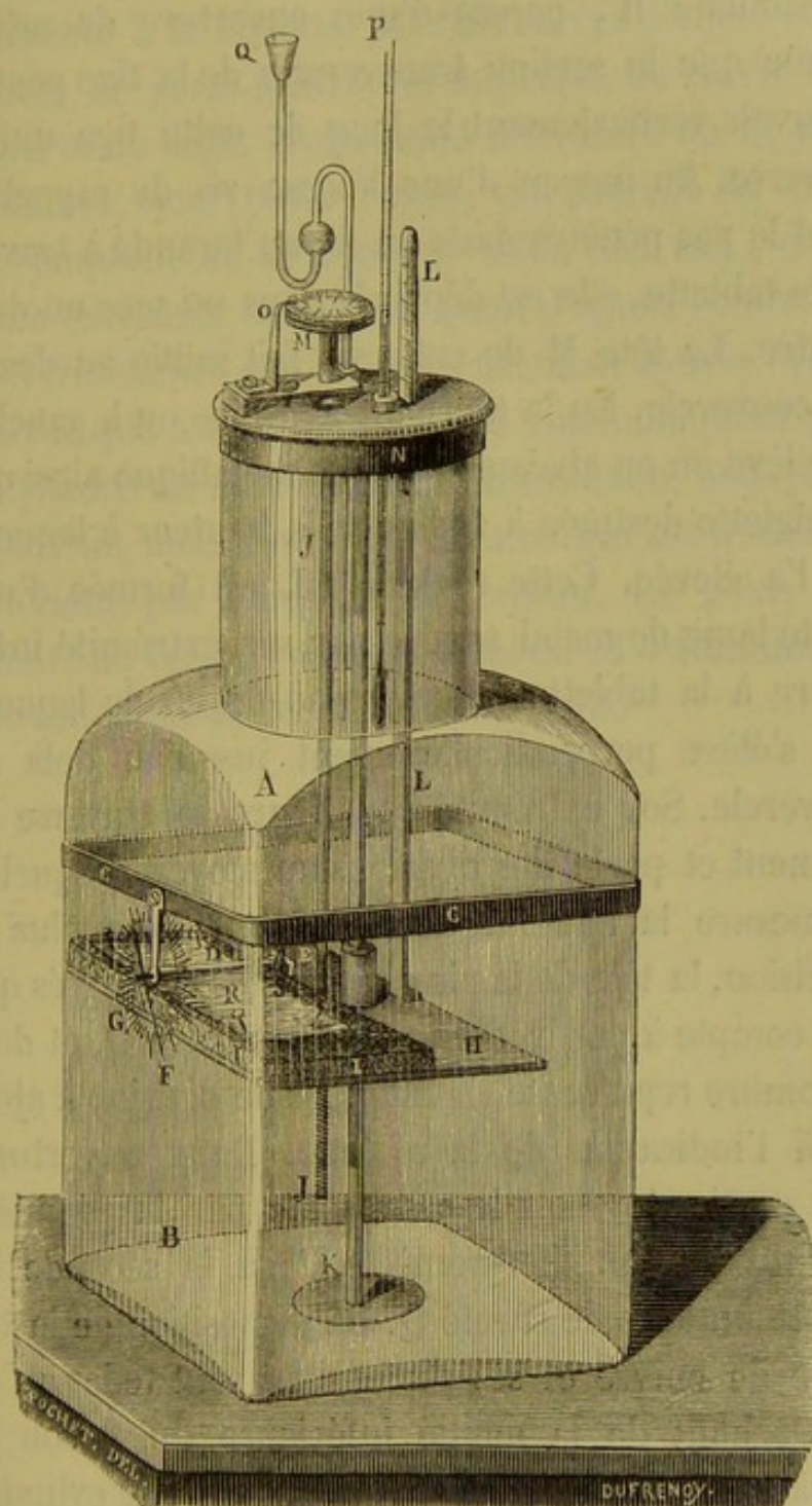
Fig. 32. — Appareil de M. Calliborcès pour mesurer les variations d'intensité des mouvements vibratiles.
