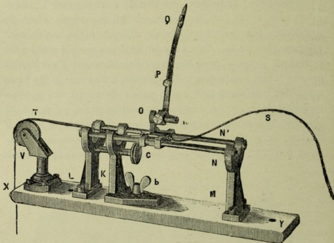
Fig. 66. — Curseur enregistreur de l'ergographe de Mosso. La corde S est attachée à la 3 e phalange du médus; à la corde T est suspendu le poids. La plume PQ écrit sur un cylindre tournant.
