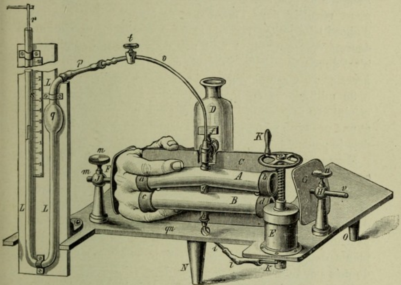
Fig. 38. — Sphygmomanomètre de Mosso.
