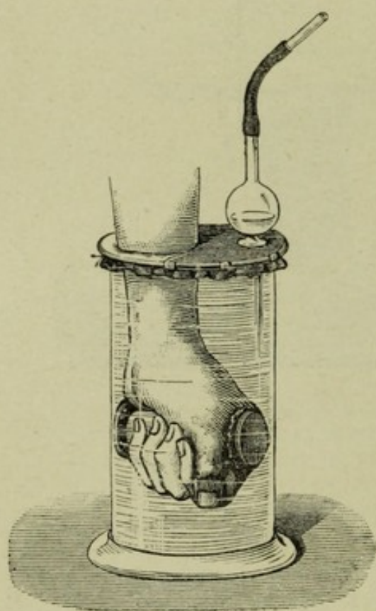
Fig. 16. — Appareil volumétrique de François-Franck.
