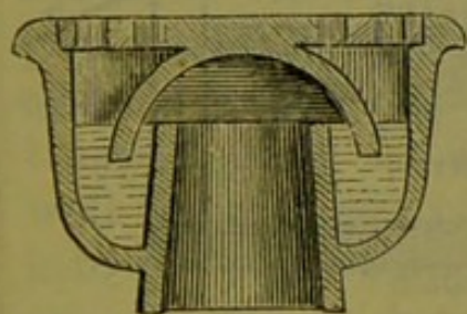
Fig. 14.—Bell Trap.
