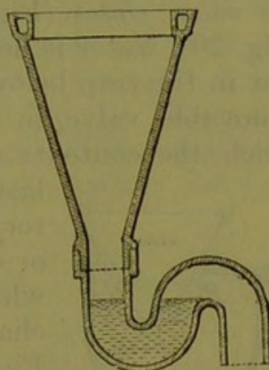
Fig. 19.—Long Hopper Closet.
