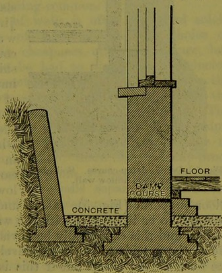
Fig. 5.—Damp-course.
