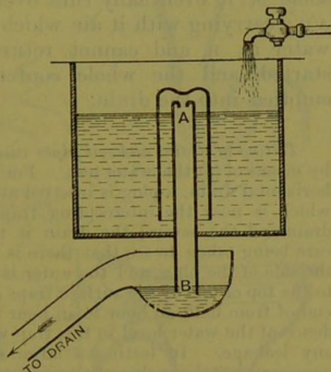
Fig. 17.—Flush-tank.
