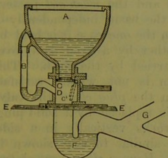
Fig. 18.—Valve Closet.
