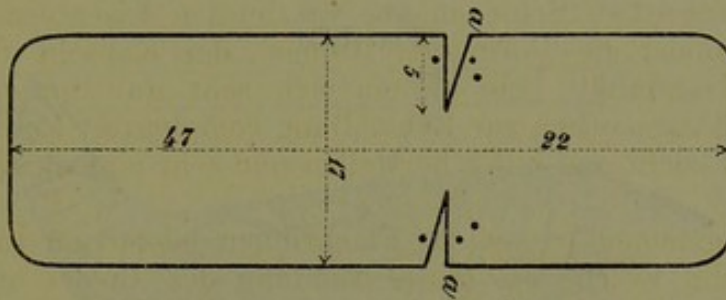
Muster zum Ausschneiden einer Armrinne nach Schoen.
