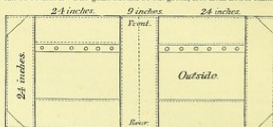
FIG. 38.—Exterior view of aparejo.—[GRANT.]
