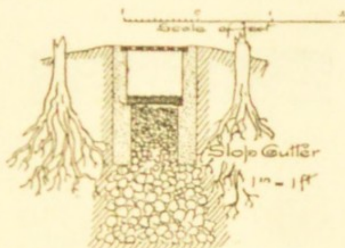
FIG. 26.—FILTRATION GUTTER.
