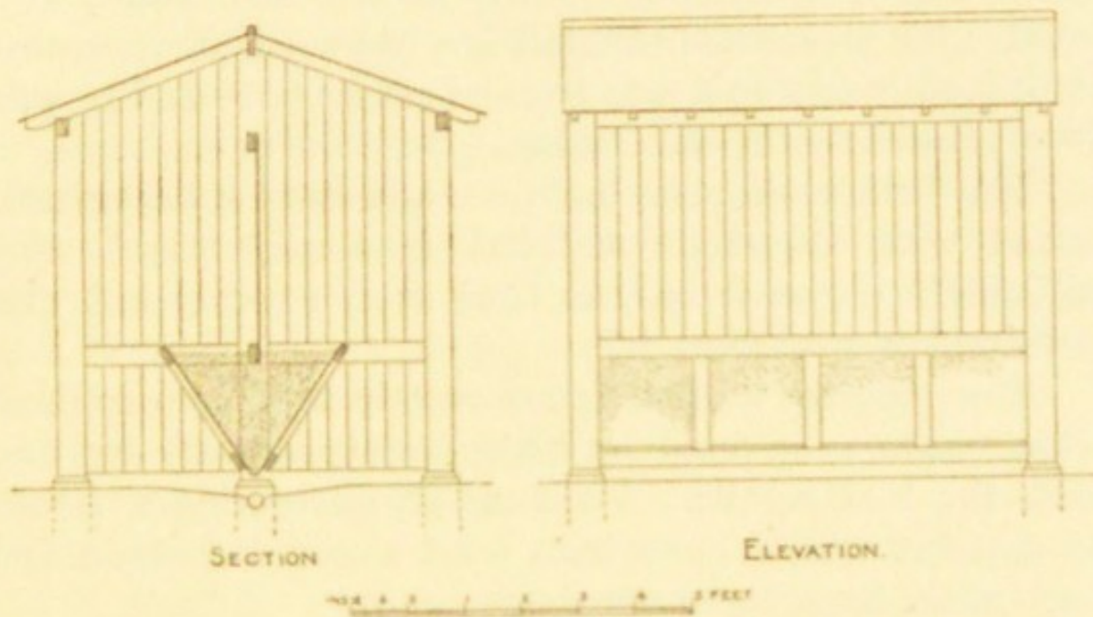
FIG. 21.—DRY URINAL.
