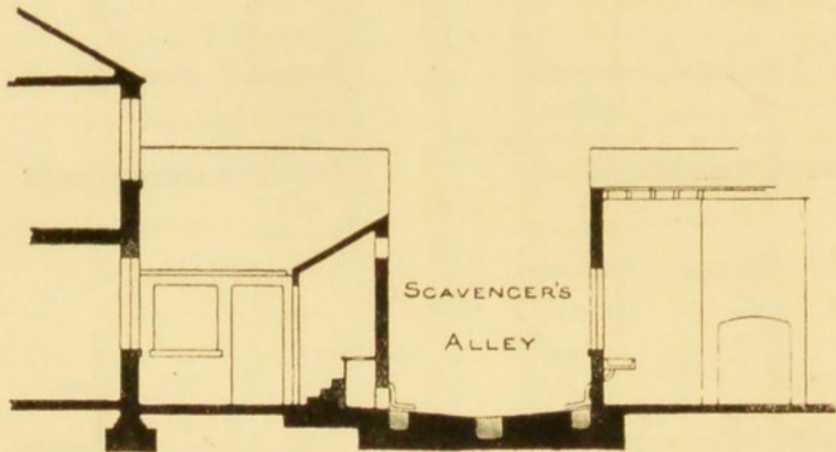
FIG. 30.—SECTION A-A.
