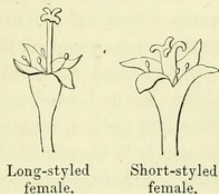
RHAMNUS CATHARTICUS.
