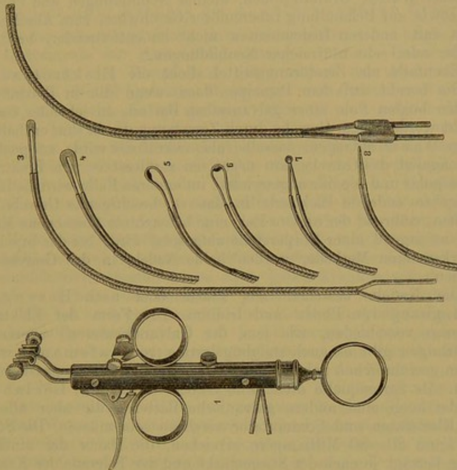
Fig. 21. Universalhandgriff des Verfassers mit verschiedenen Brennern.
