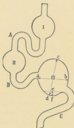
Rückflußrohr nach Cathcart.
