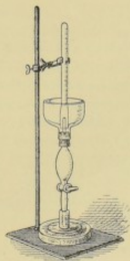
Apparat für die Bestimmung des Harnstoffs nach Knop-Hüfner.
