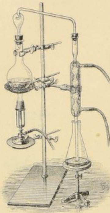
Apparat für die Ammoniakdestillation mit Wasserkühlung.
