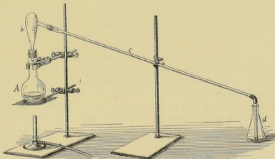
Apparat für die Ammoniakdestillation mit Luftkühlung.
