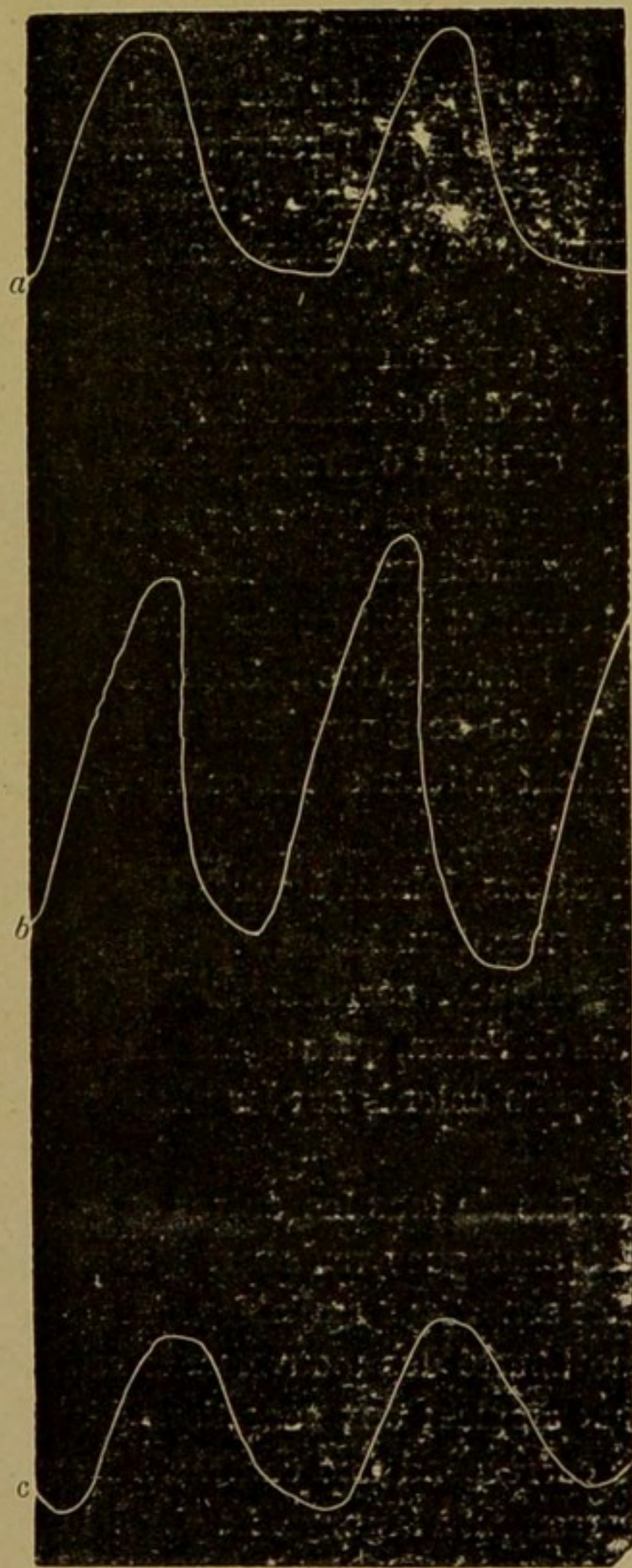
Fig. 4. — Courbes de la respiration chez C. : a , à l'état normal; — b , à l'éclairage rouge; — c , à l'éclairage bleu.
