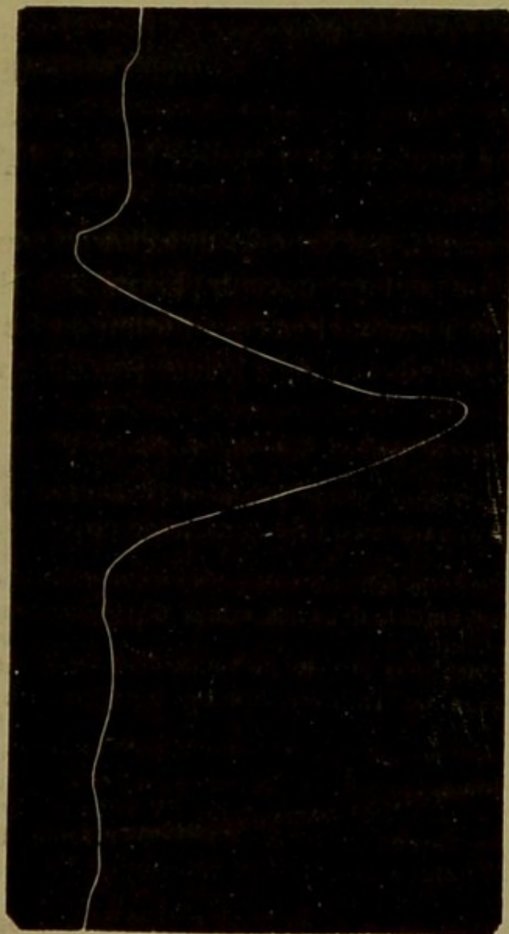
Fig. 21. — Trace phethismographique montrant la diminution de volume de la main droite et de l'avant-bras au moment où, le sujet étant placé sur le tabouret de la machine statique, on décharge la machine.
