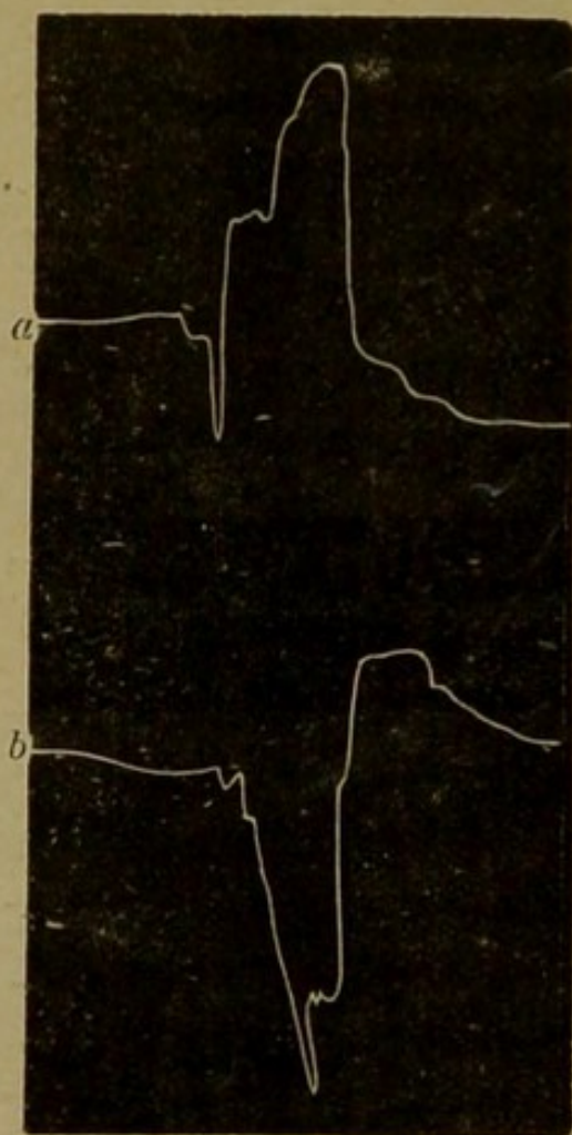
Fig. 14. — Reaction musculaire chez B., sous l'influence d'une hallucination pénible (un hibou sur la fenêtre). — a , courbe du long supinateur; — b , courbe du jumeau externe.
