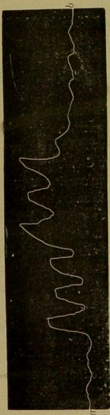
Fig. 7. — Modification du pouls huméral (a-b), sous l'influence d'une excitation par la lumière rouge.
