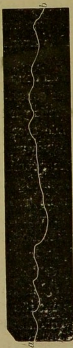
Fig. 8. — Modification du pouls huméral sous l'influence de l'obscurité (a-b).
