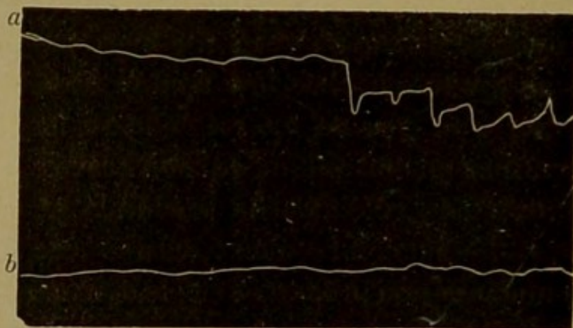
Fig. 1. — Réactions musculaires chez G. : a , courbe du long supinateur droit qui subit des excitations au degré 7 de l'échelle Dubois-Raymond (7-5), puis au degré 5 (5-5); — b , muscle long supinateur gauche qui commence à éprouver des ondulations quand les excitations sont à 5.
