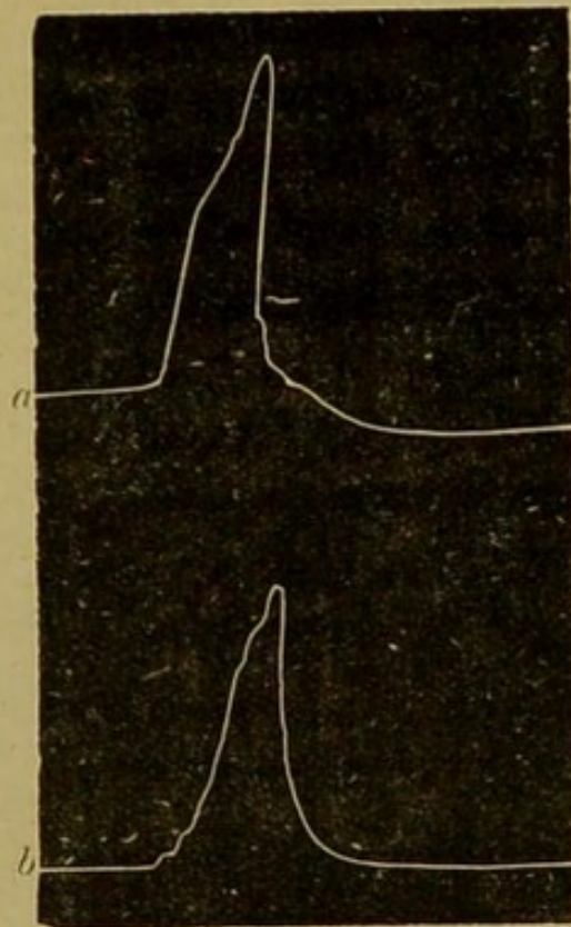
Fig. 10. — Réaction musculaire chez C., sous l'influence d'une courte excitation par le vert. a , tracé du long supinateur droit; — b , tracé du jumeau externe droit.
