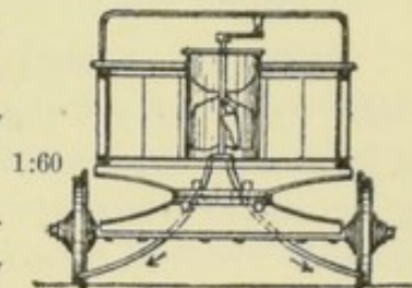
FIG. 163.—SALT SPRINKLER.
