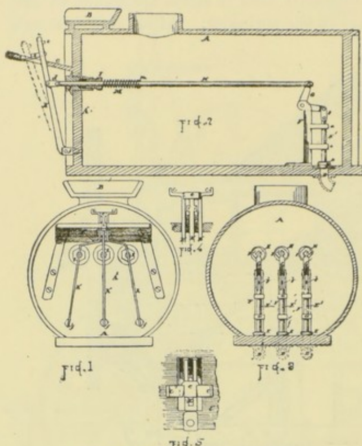
FIG. 217.—MONITOR SPRINKLER.
