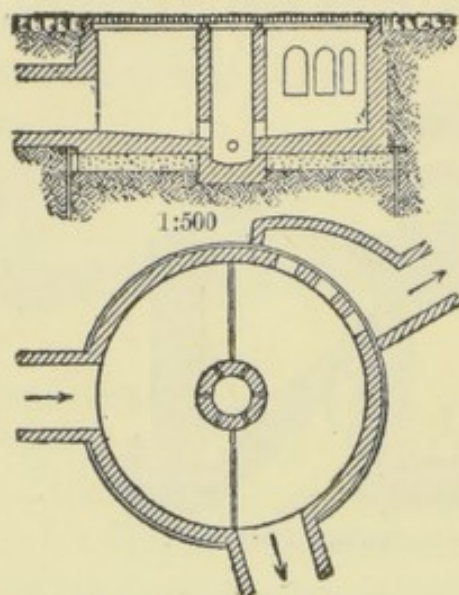
FIG. 130.—SAND PIT.
