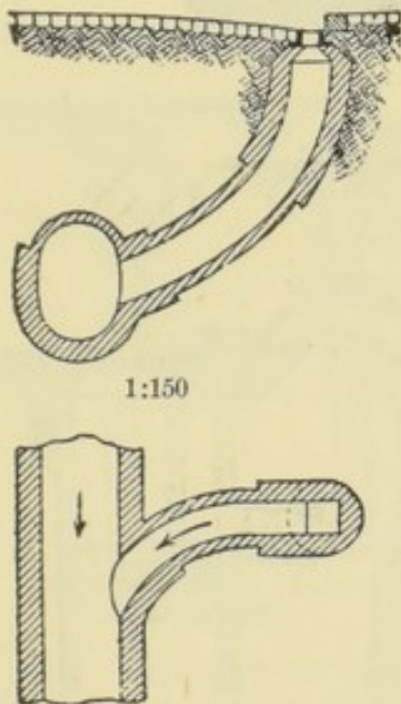
FIG. 59.—STREET INLET, HAMBURG.
