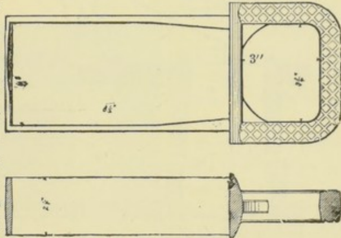
FIG. 207a.—MANHOLE STEP.
