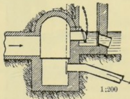
FIG. 54.—OUTLET AT DANZIG.
