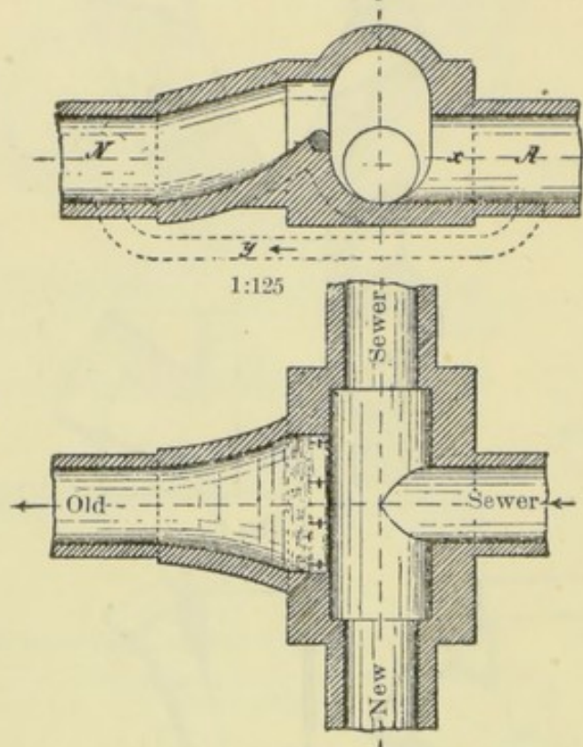
FIG. 43.—RELIEF OUTLET, LONDON.
