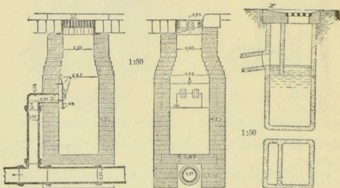
FIG. 63.—STREET INLET, BERLIN.
