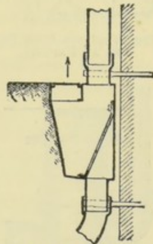
FIG. 76.—RAIN PIPE IN-LET, KARLSRUHE.
