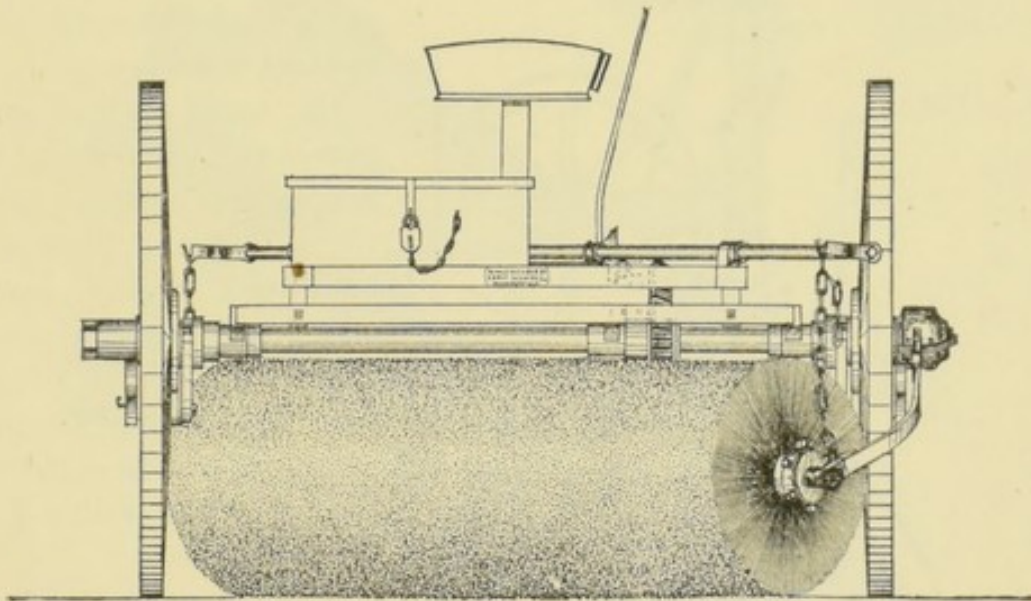
FIG. 214.—STREET SWEEPER, PROVIDENCE, R. I.
