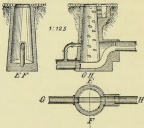
FIG. 84.—FLUSHING SHAFT AT WIESBADEN.
