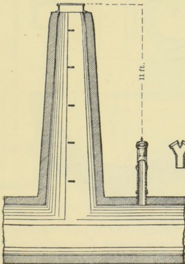
FIG. 205.—MANHOLE ON DEEP SEWER.
