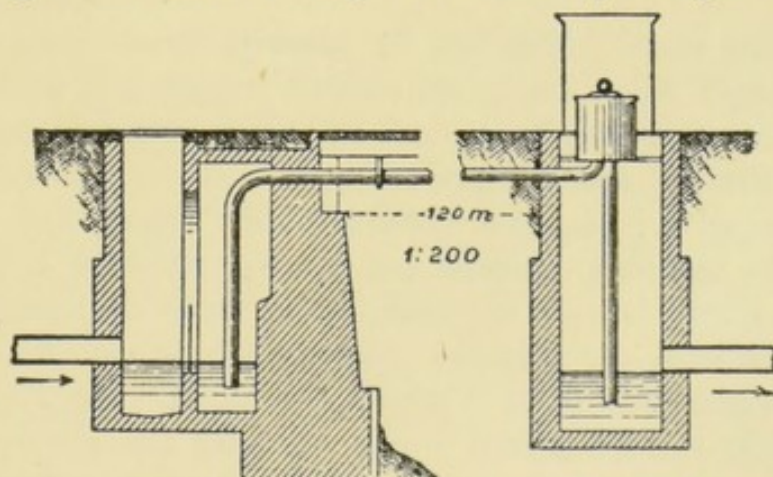
FIG. 57.—SIPHON IN BRESLAU.
