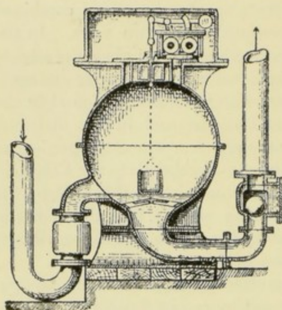
FIG. 124.—SHONE EJECTOR.
