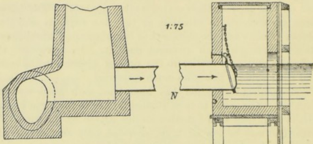
FIG. 113.—OUTLET AT DANZIG.
