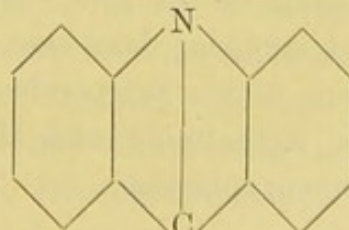
Acridin.
