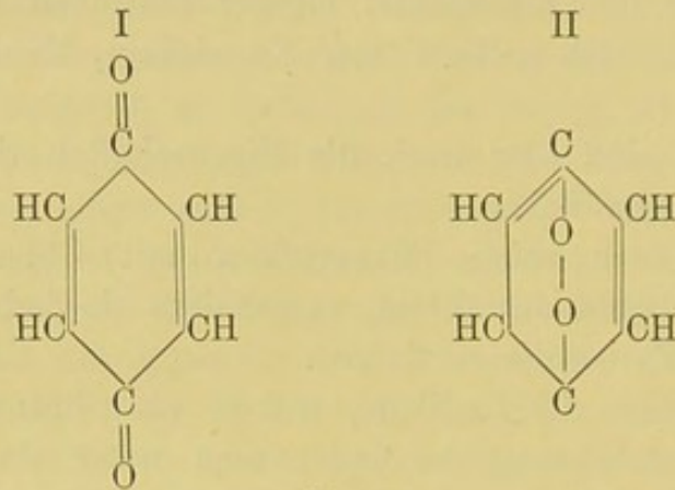
Chinon.
