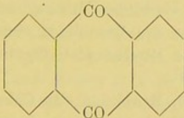
Anthrachinon.
