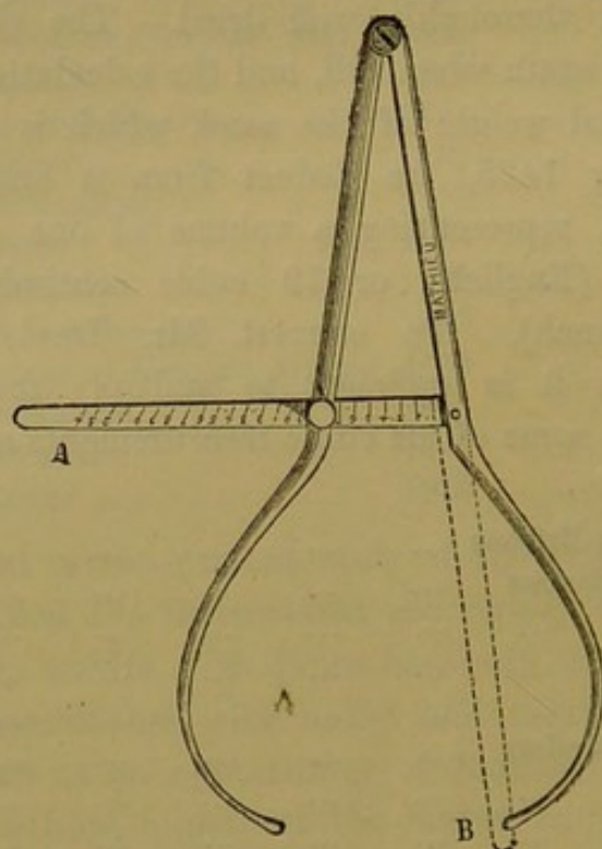
FIG. 26.—The Callipers (Compas d'Épaisseur).
