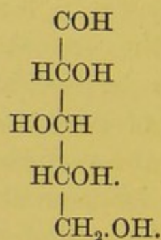
l. xylose.
