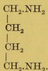
Putrescin.
