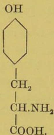
Tyrosin.
