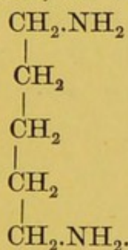
Cadaverin.
