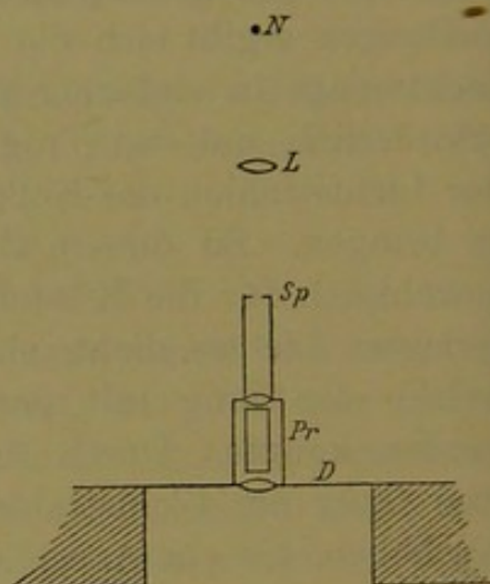
Fig. 1. Anordnung der Bleichungsversuche.
