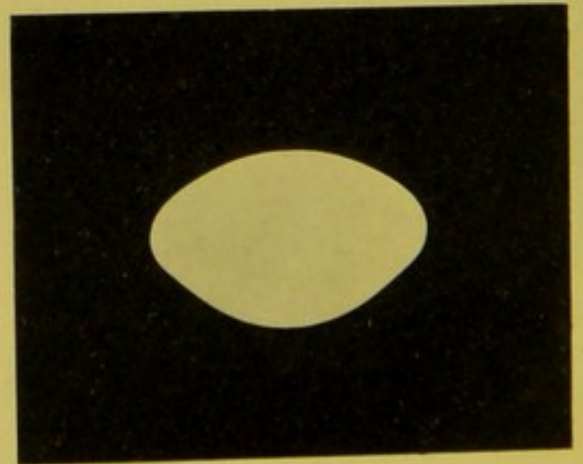
Schema der Linse der Taube.
