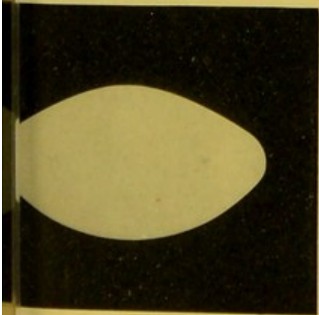
Schema der Linse des Affen.
