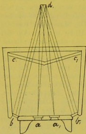
Fig. 26. Pseudoskop von Bertin-Sans.
