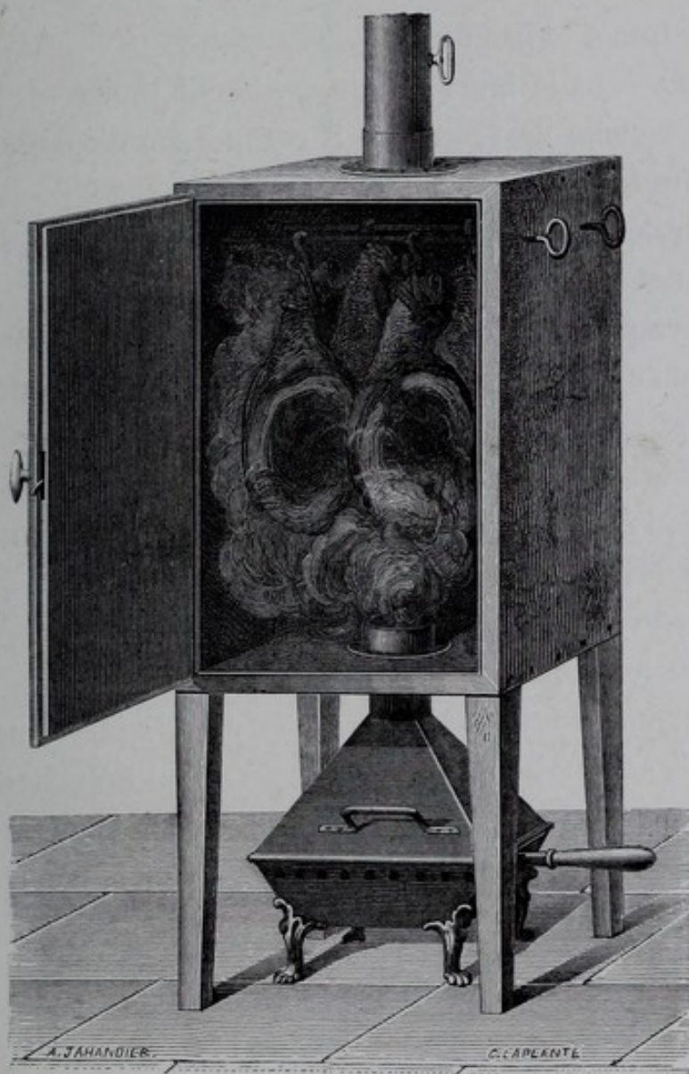
Fig. 2. — Boîte à fumer.
