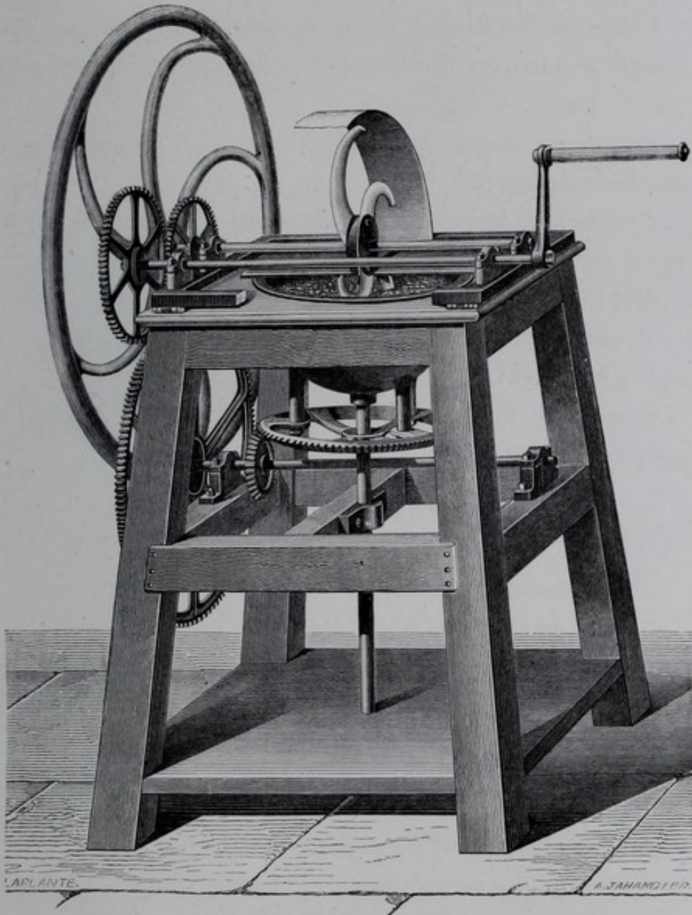
Fig. 11. — Machine à hacher.
