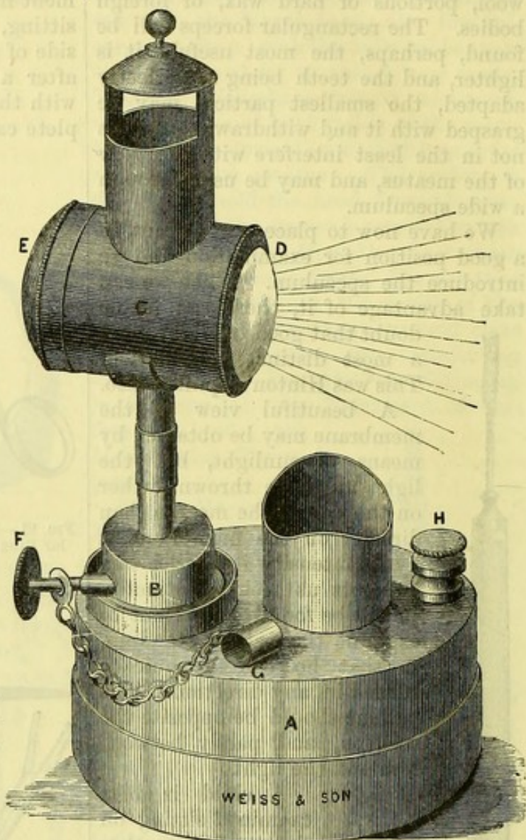
FIG. 26. — Portable Lamp.
