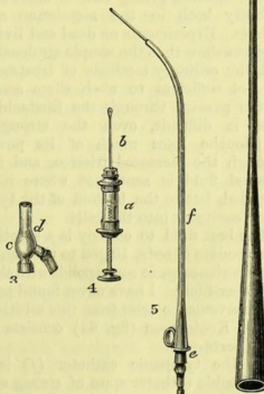
FIG. 64.—Koniontron.
