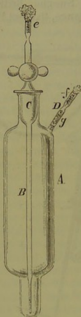
Fig. 20. — Appareil de Straus et Wurtz pour compter les germes de l'air en faisant barboter ce dernier dans la gélatine. — A, tube dans lequel est enfermée la gélatine; e, C, B, bouchon tubulé qui donne accès à l'air chargé de germes; D, tube d'aspiration.
