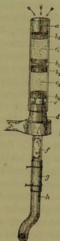
Fig. 30. — Appareil de Pétri pour l'analyse bactériologique de l'air. — L'air pénètre suivant la direction des flèches en a ; c 1 , c 2 , sable fin; b 1 , b 2 , b 3 , b 4 , disques treillagés de fil de fer; f , ouate; g , h , tube qui conduit l'air à une pompe.
