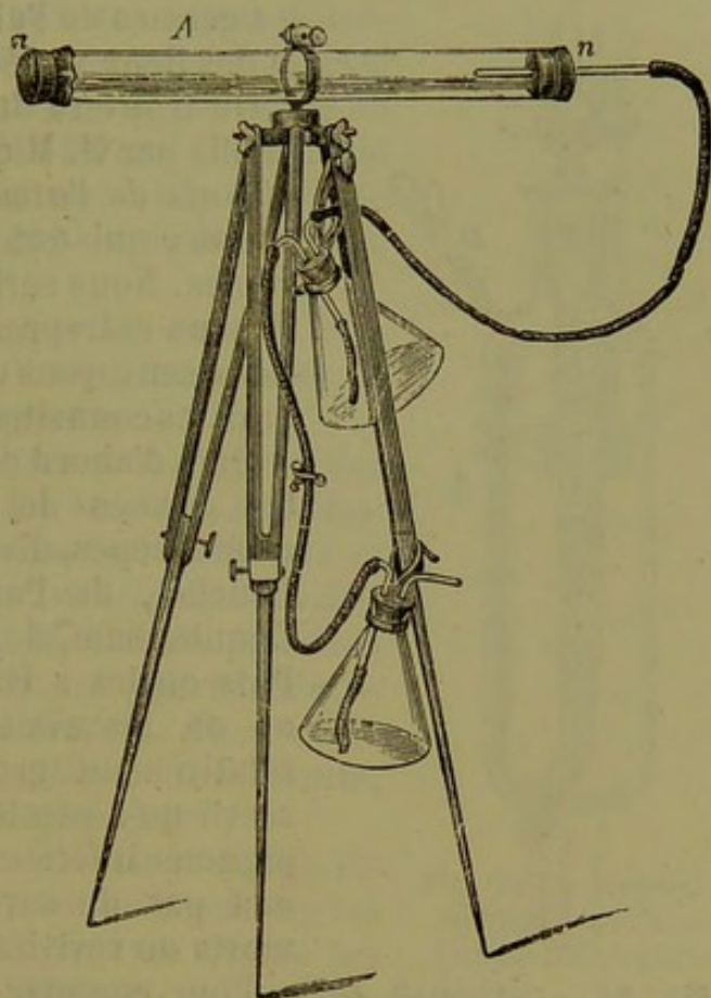
Fig. 28. — Appareil de Hesse pour compter et cultiver les germes de l'air. — a , membrane de caoutchouc fermant l'une des extrémités du tube A qui contient la gélatine; n , tube de verre servant à l'aspiration de l'air.
