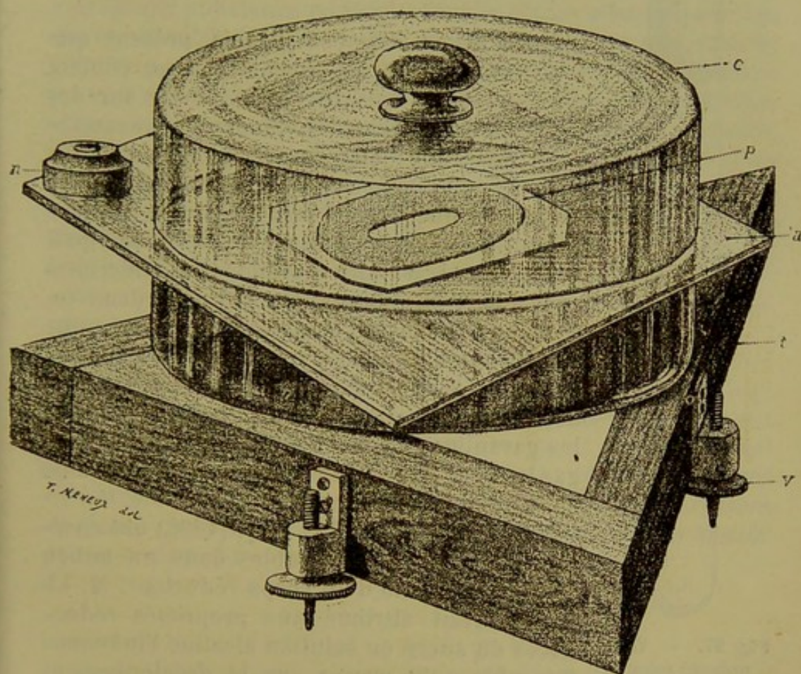
Fig. 26. — Appareil de Koch destiné à faire des cultures d'isolement sur des plaques de verre. — t , trépied, muni de vis calantes v , destiné à soutenir la plaque de verre a dans une direction horizontale; n , niveau à bulle d'air; p , plaque sur laquelle la gélatine se solidifie; c , cloche protectrice.
