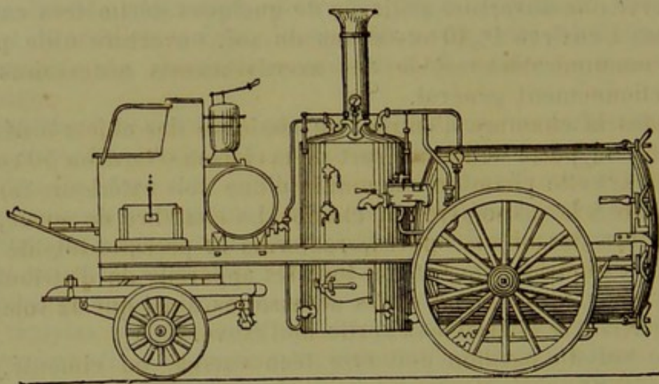
Fig. 45. — Étuve mobile de MM. Geneste et Herscher.
