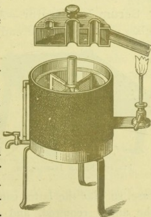
FIG. 14.—SERUM STERILISER
