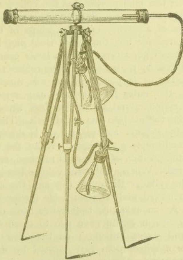
FIG. 136.—HESSE'S APPARATUS.
