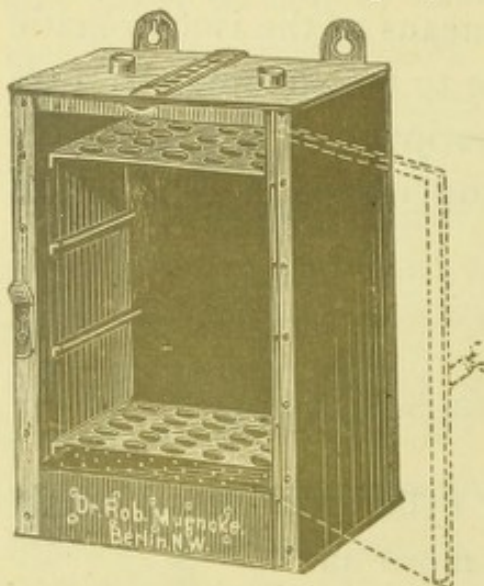
FIG. 2.—HOT-AIR STERILISER.
