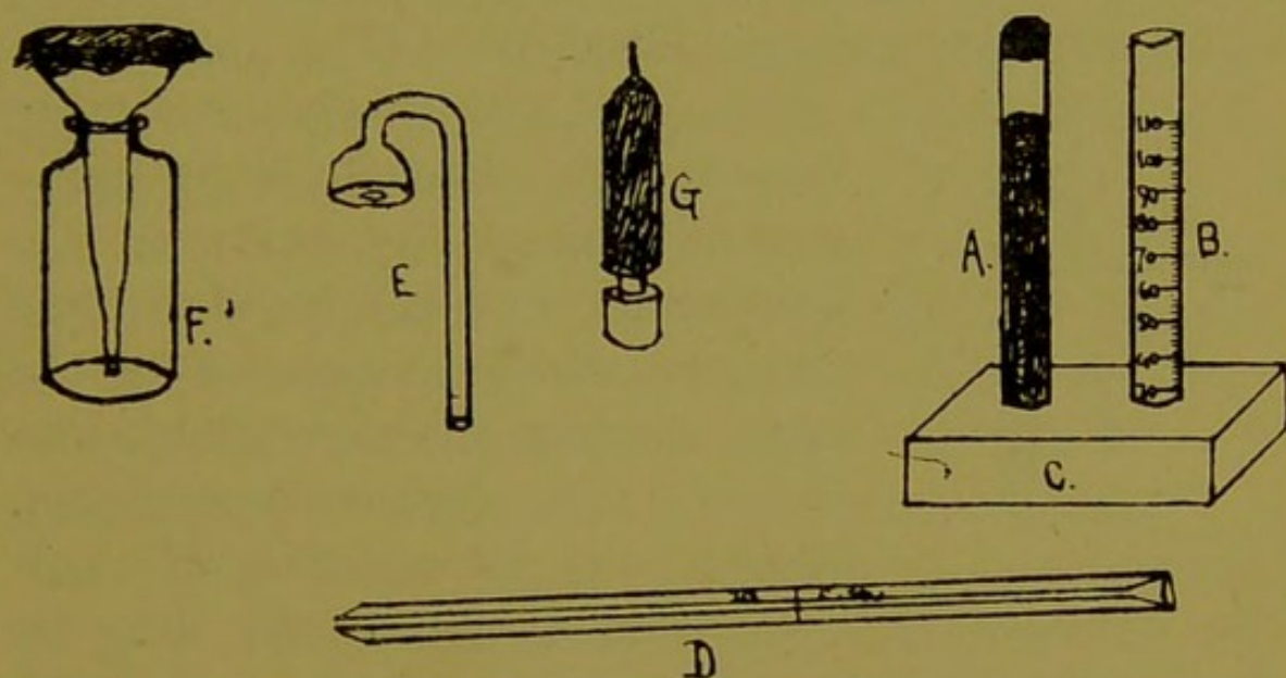
FIG. 29.—Haldane's Hæmoglobinometer.
