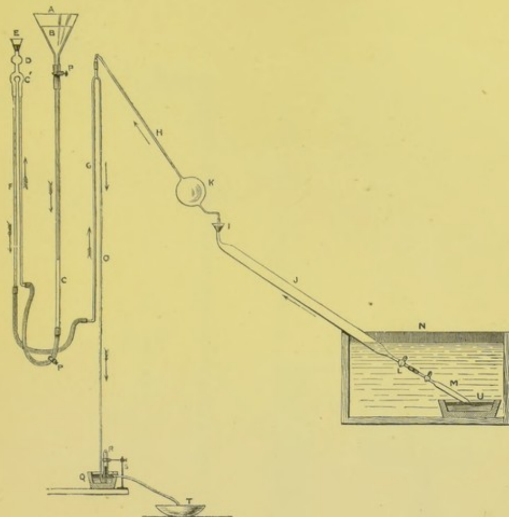
FIG. 199.—Frankland-Sprengel pump (§ 26).
