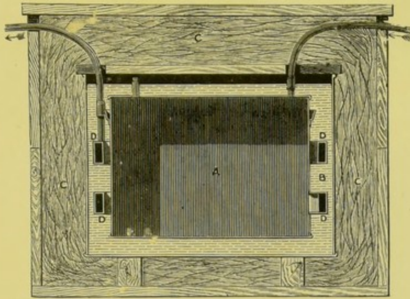
FIG. 265.—The calorimeter (§ 116).
