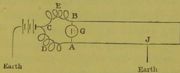
Fig. 490.—Loop Test.
