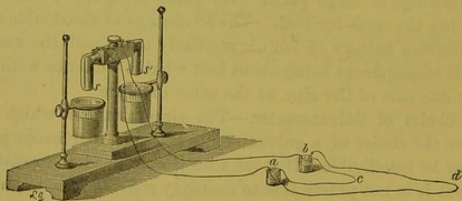
Fig. 483.—Divided Circuit.
