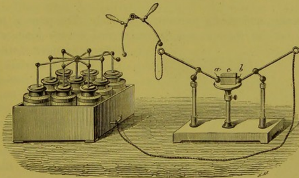
Fig. 393.—Universal Discharger.
