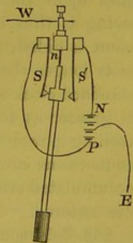
Fig. 582.—Controlling Pendulum.
