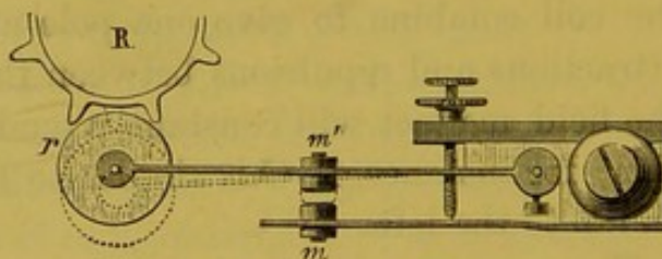
Fig. 581.—Distributor.
