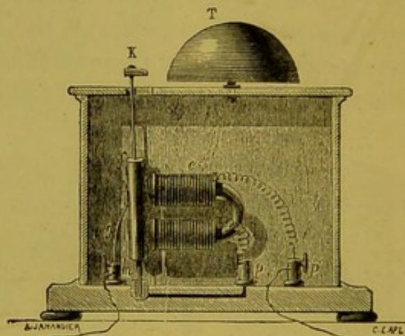
Fig. 565.—Vibrating Alarum.
