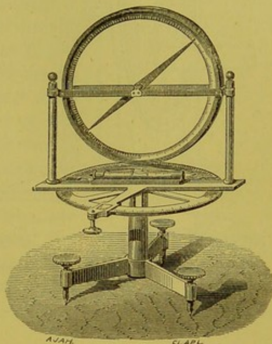
Fig. 427.—Dip-circle.
