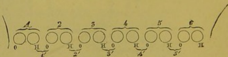
Fig. 473.—Grotthius' Hypothesis.
