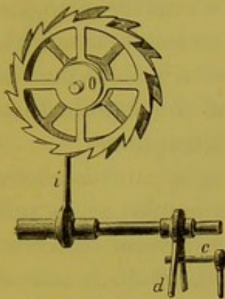
Fig. 563.—Escapement.
