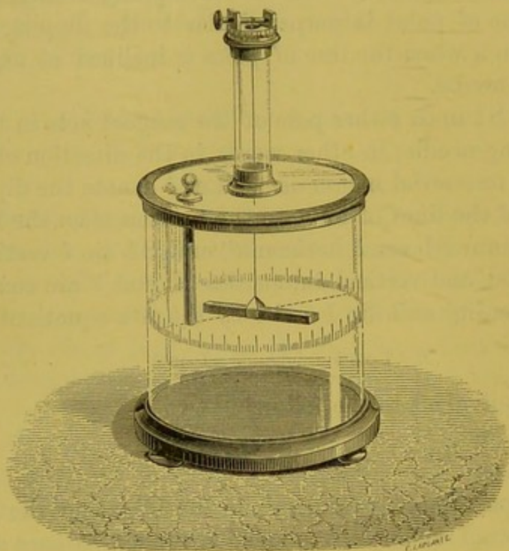
Fig. 424.—Torsion-balance.
