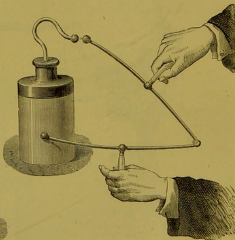
Fig. 382.—Discharge of Leyden Jar.
