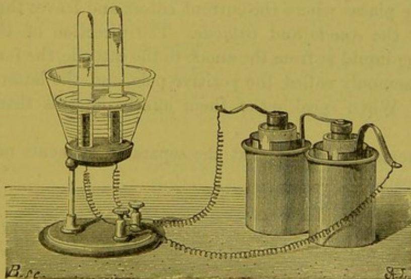
Fig. 472.—Voltmeter.
