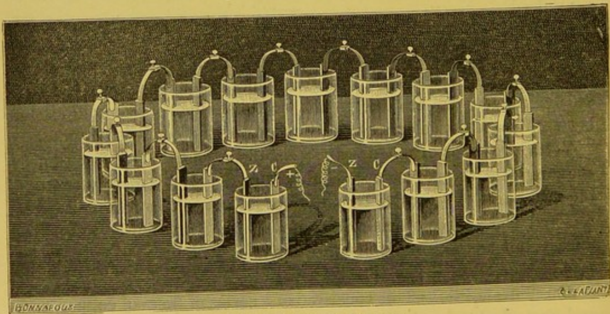
Fig. 451.—Couronne de Tasses.
