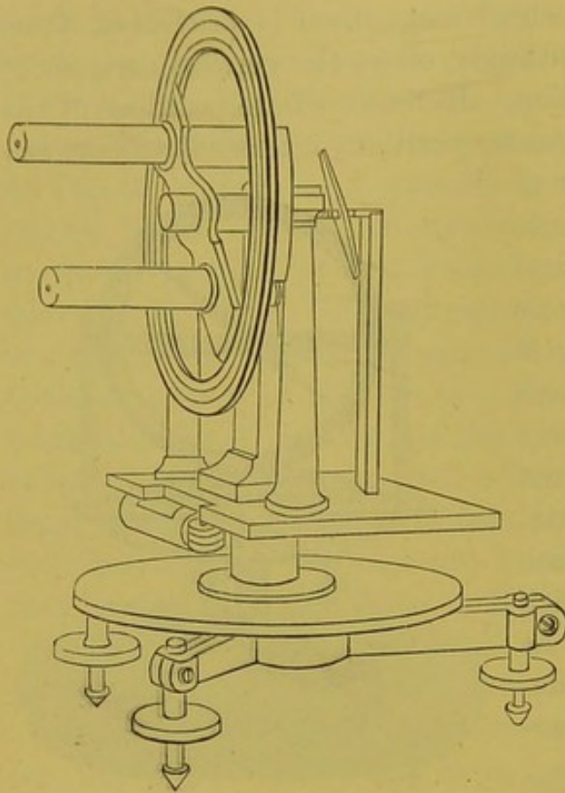
Fig. 428.—Kew Dip-circle.
